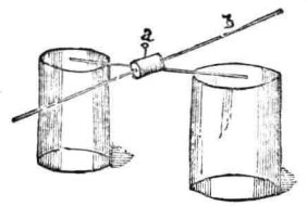
磁傾角圖
