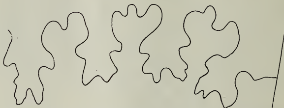
Fig. 7. Teilung des Aussenlobus bei 10 mm Windungsradius. \frac{15}{1} .
