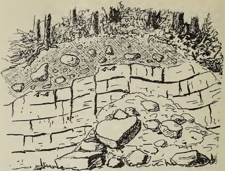
Fig. 7. Steinbruch (C) am Nordfuß des Ziegelberges; verruselte Tenuilobatuskalke von überschobener Masse überlagert; s-s Schließflächen.
