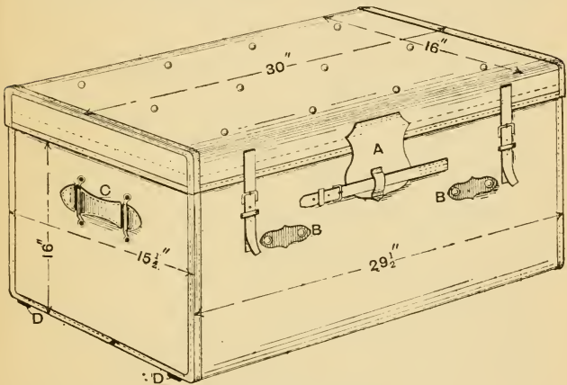
Fig. 95.—Imperial Trunk.
