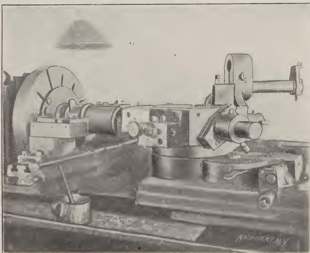
Fig. 26. Turning Cylinders
