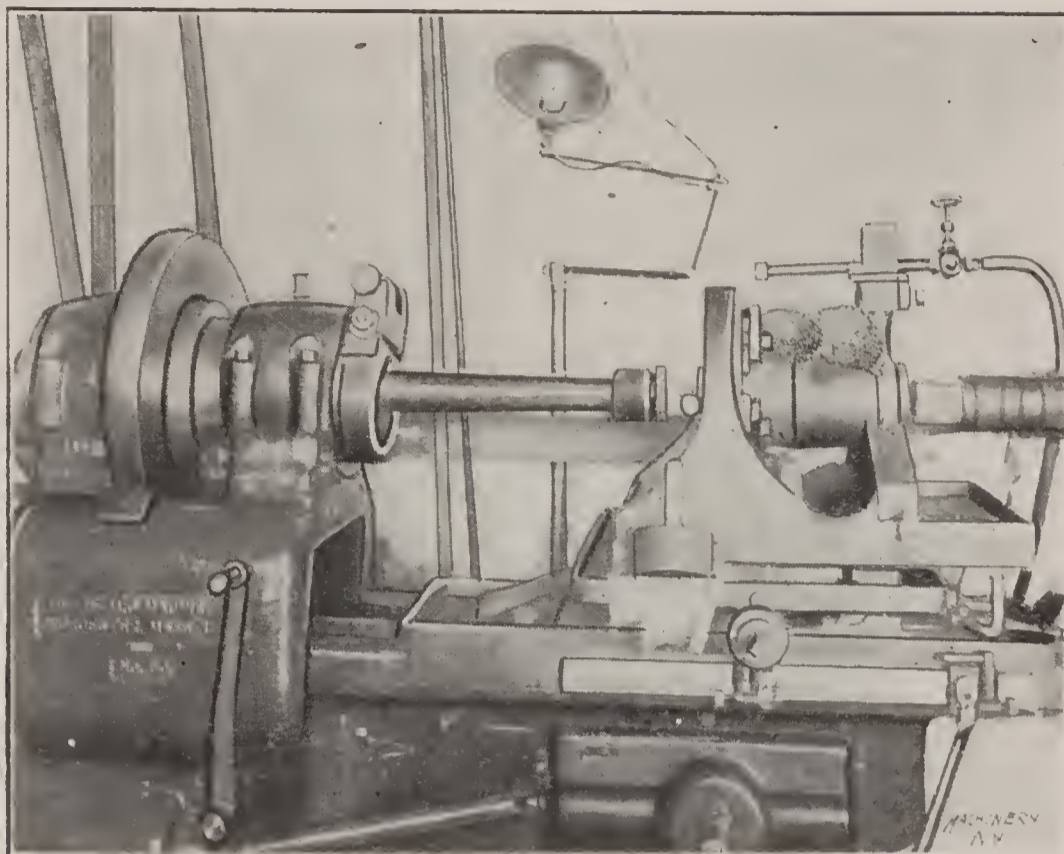
Fig. 27. Grinding Cylinders
