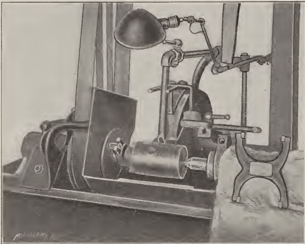
Fig. 29. Grinding Pistons
