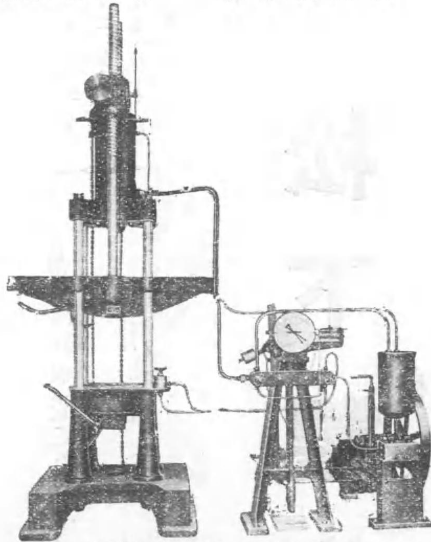
油圧式 50 吨萬能材料試験機 Type A, No. 50 ABCT
