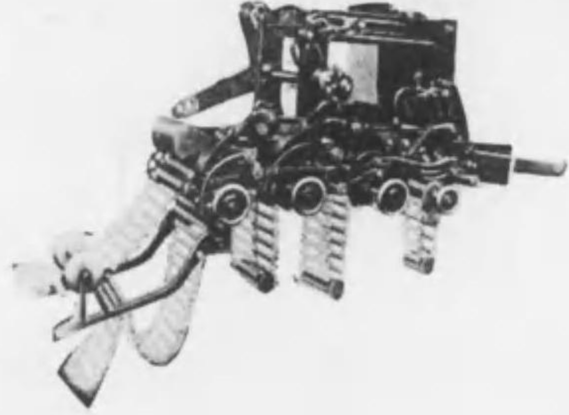
三本シリンダードビー装置
