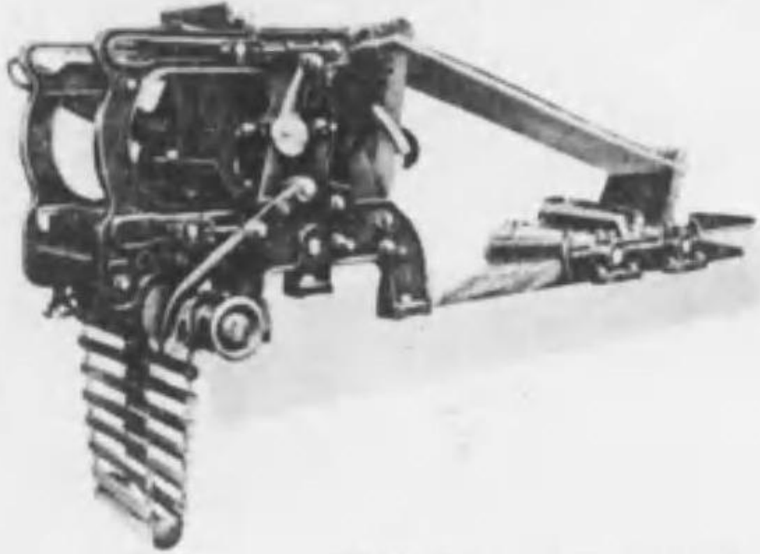
ダブルリフトシングルシリンダードビー
