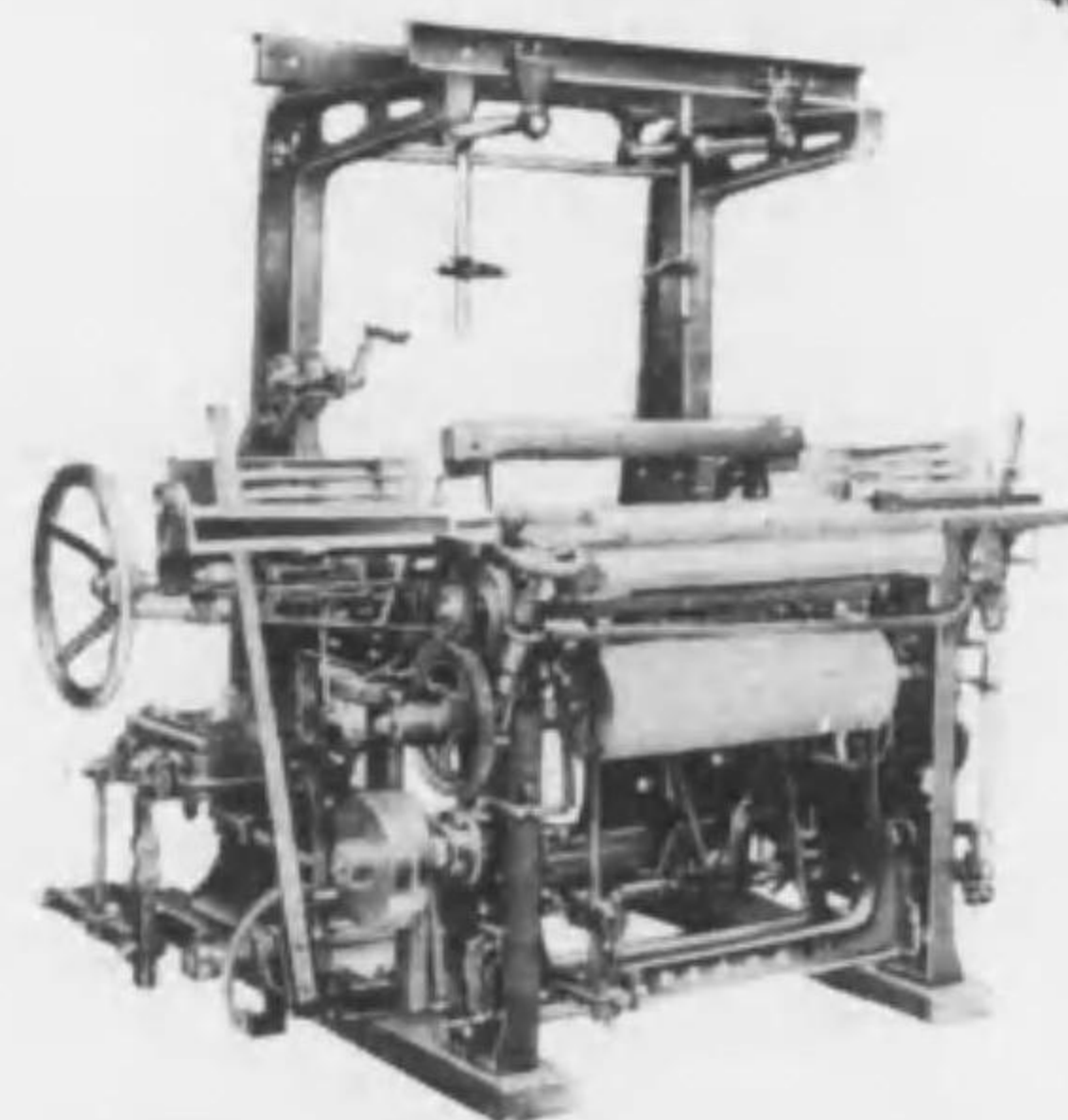
兩側四丁絹布力織機
