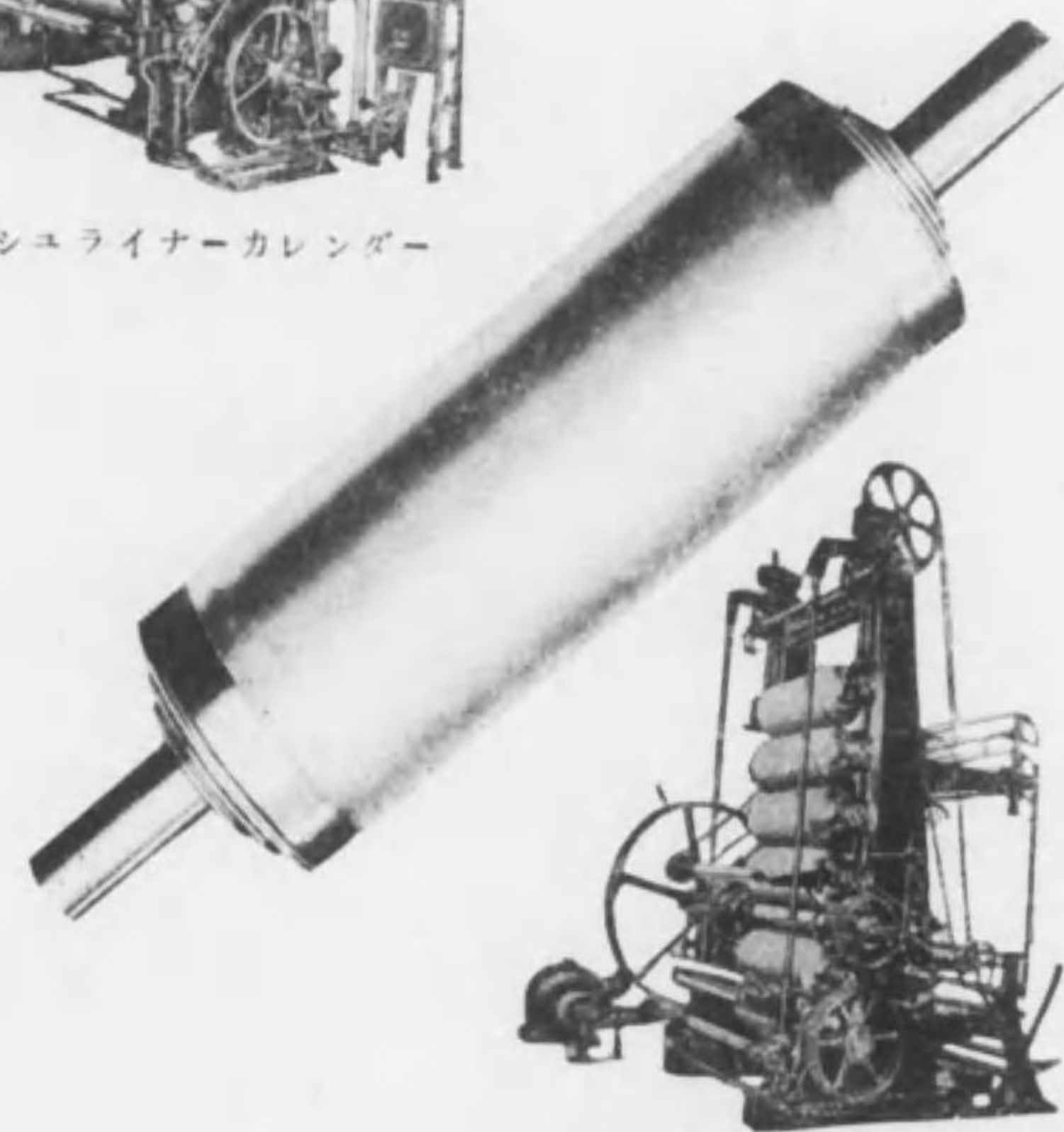
七本ロール製出機(C型)
