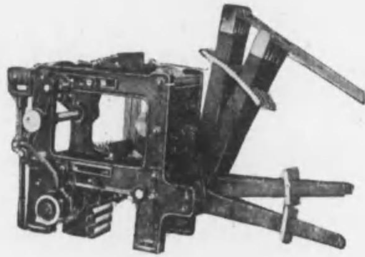
毛織用四巾ドビー装置
