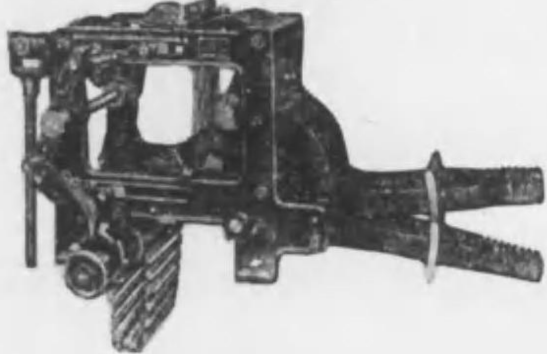
ダブルリフトシングルシリンダードビー
