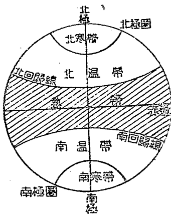
地球五帶圖
