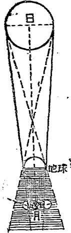
月蝕
