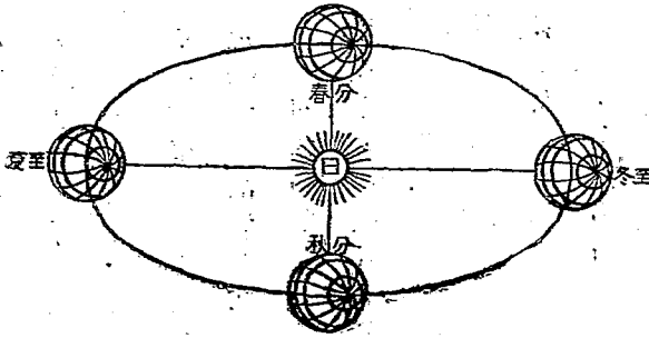
地球公轉圖
