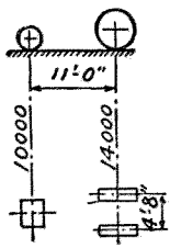
十二噸壓路機
