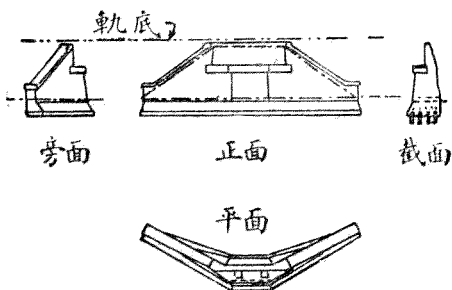
第四十六圖 雙翼橋座
