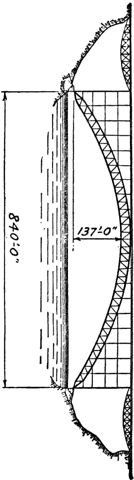
第十六圖 美國耐亞嘎拉河上之耐亞嘎拉克力夫脊公路橋
