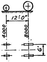
六噸貨車
