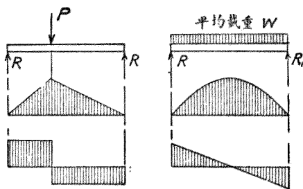
第三十一圖 撓曲力及剪割力之分配圖
