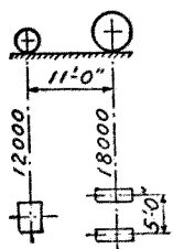
十五噸壓路機
