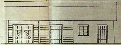
Хозяйствен. постройки Фасадъ здан. В
