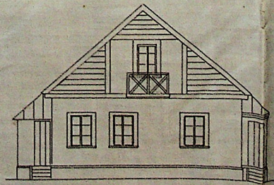
Зд. Г Фасадъ
