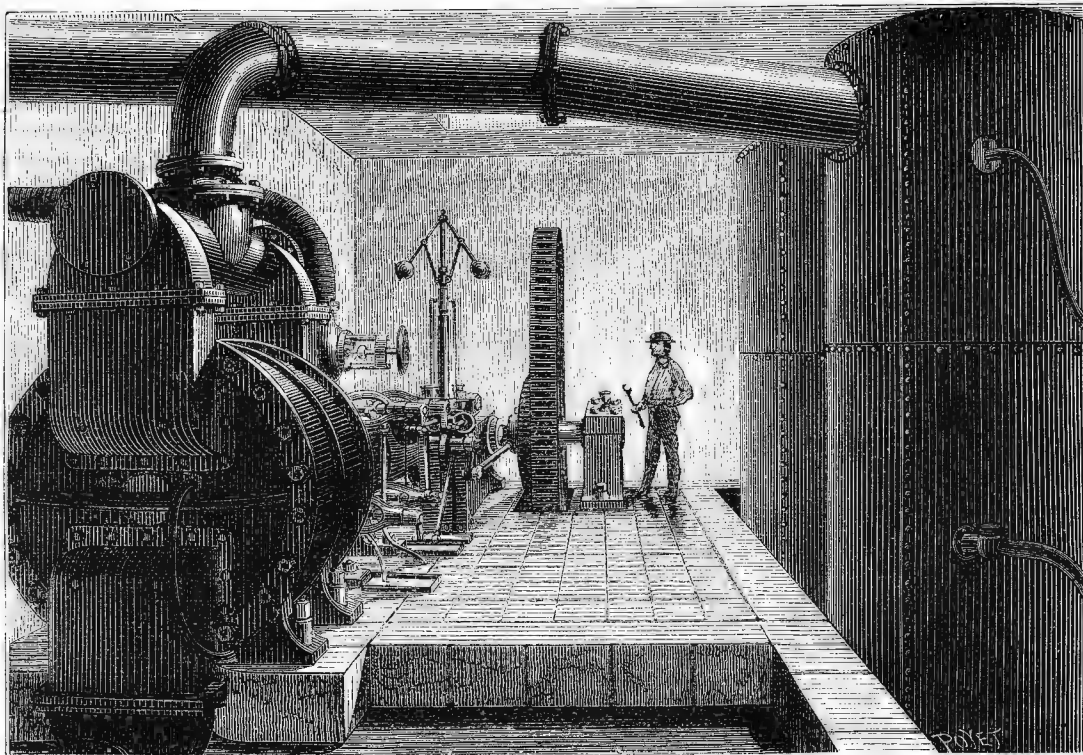
Распределение силы. Фиг. 1. Центральный заводъ.
