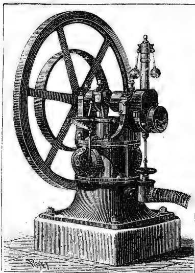
Распределение силы. Фиг. 2. Двигатель разрѣженнымъ воздухомъ.
