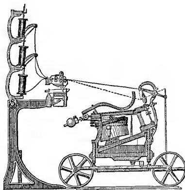
MULE SPINNER.
