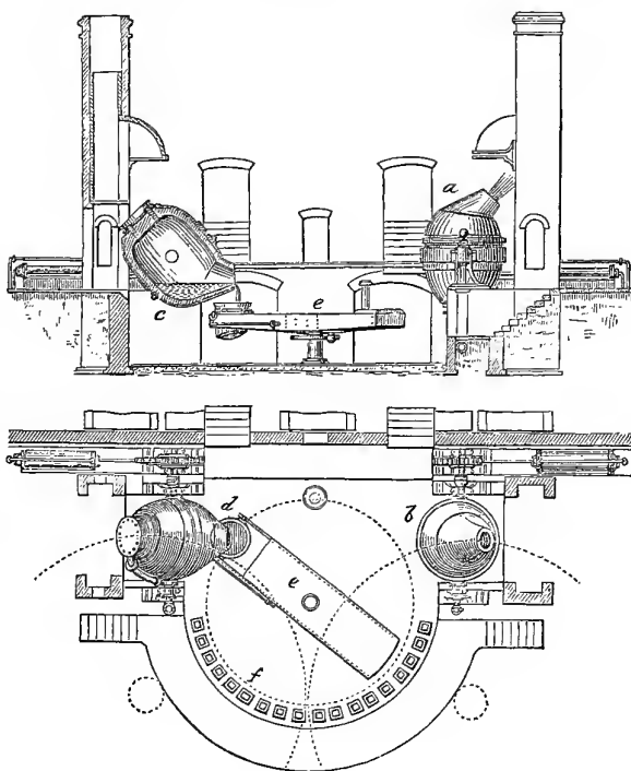
BESSEMER PLANT.
