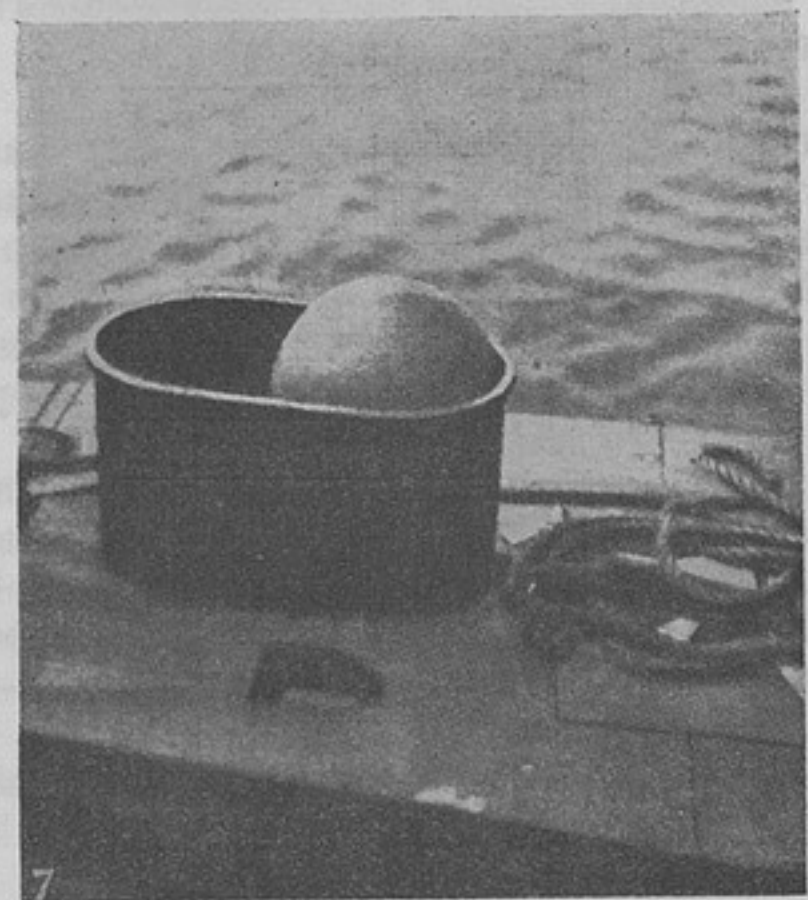
Спасеніе затонувшихъ въ подводной лодкѣ. Шаръ-буксъ автоматически выбрасывается на поверхность, обозначая мѣсто гибели лодки.
