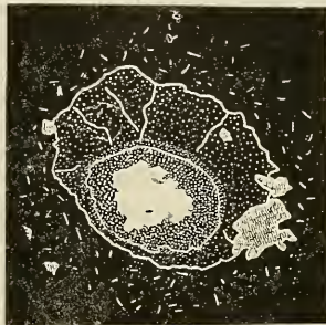
Fig. 5. Gediegenes Eisen in Magnetit eingewachsen, in diesem Relikte von Magnetkies. Vergr. 214.
