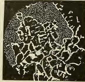
Fig. 2. Rekristallisationsstrukturen in pseudomorpher Magnetkiesknolle. Vergr. 53.
