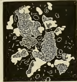
Fig. 1. Magnetkiesknolle mit gediegenem Eisen, Quarz in korrodierten Körnern mit Augit- und Glas-Kränzchen. Vergr. 120.
