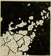
Fig. 3. Endigung einer Pyritnase im Basaltjaspis, noch nicht in Magnetkies umgewandelt. Vergr. 31.
