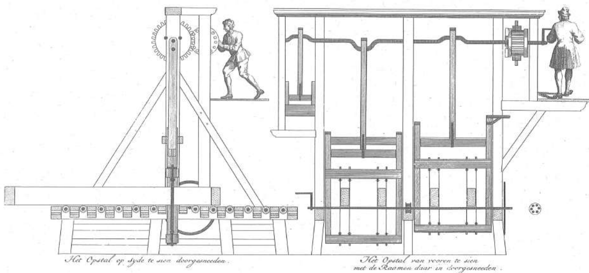
De Hee stelling in de gronde met syn Rollen en de Hee daar booven op liggende.
