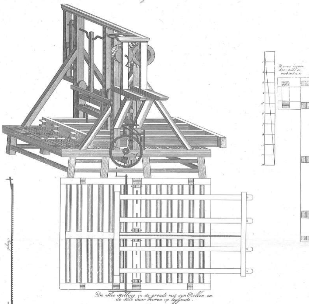
Opstal in 't verscliet van een Schryn werkers Plaat Moolen.
