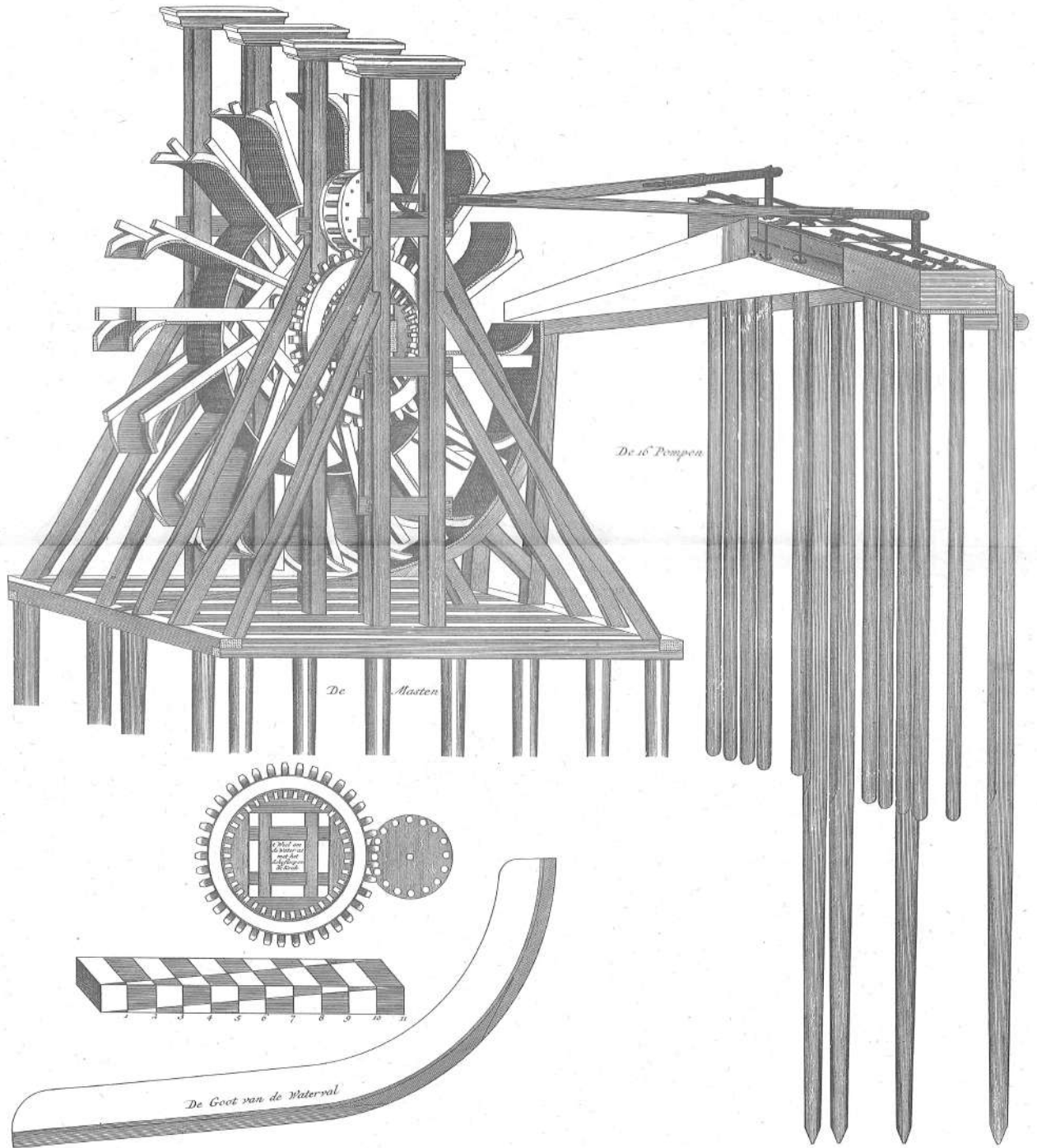
Den Opstal van een van selfs gaande Pomp Molen in het verschie.
