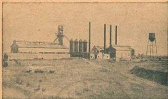
圖九 龍烟鐵礦公司 在 北平西郊石景山 所建 煉鐵廠 ，足見其 原定計劃 的規模。
