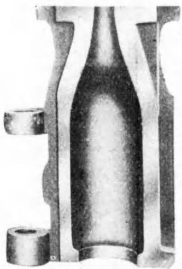
硝子瓶金型 型金瓶油醬酒
