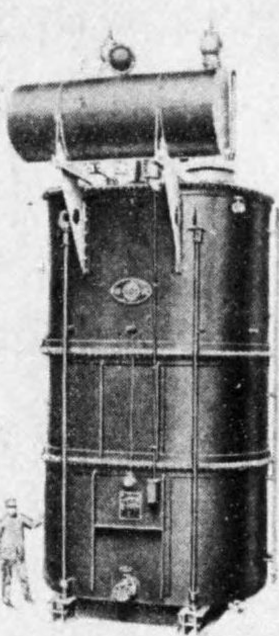
18333kVA水冷式變壓器
