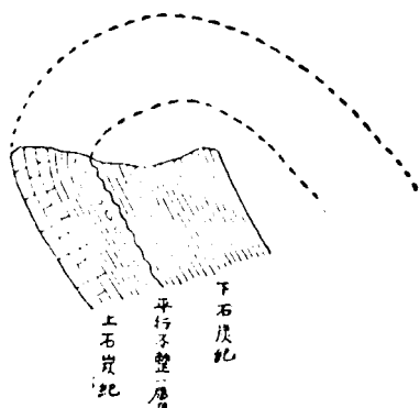
雲南東南部地質剖面圖 第二圖
