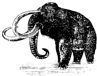
第一圖 猛 獁 象
