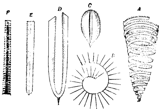
第九圖 筆石
