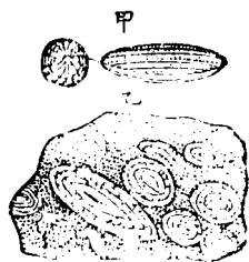
第五圖 鮫石蟲的種類 甲) 出石中的取出面 乙) 鮫石的面
