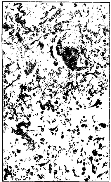
第 二十 圖 三 葉 蟲 石 化
