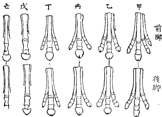
圖三第 馬的足進的化
