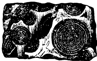
第四圖 貨幣蟲的化石
