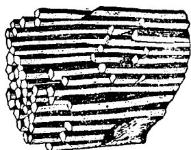
珊瑚窩蜂的紀留志下 圖七第
