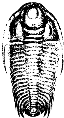
第 十 一 圖 兜頭蟲 寒武紀的三葉蟲類
