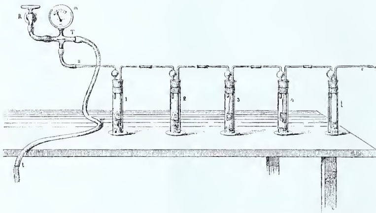
FIG. 4. — Appareil disposé pour une série de cultures dans de l'air privé de germes, constamment renouvelé. — R, robinet par où rentre l'eau; T, trompe de Brewer; l, tube par où l'eau s'écoule; l'air, appelé par la trompe, passe en c à travers du coton roussi, traverse le flacon laveur l, puis passe dans des cultures successives 5, 3, 2, 1; m, manomètre.
