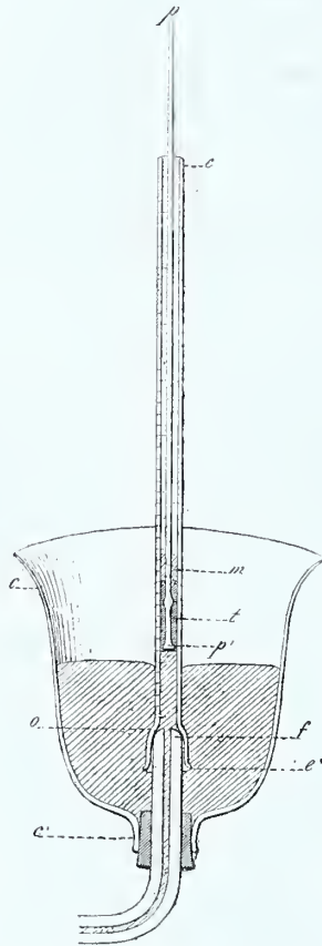
FIG. 1. — Éprouvette graduée à piston, placée sur la cuvette à mercure de la pompe d'Alvergniat. — ec' , tube gradué; pp' , tige du piston; t , corps du piston.
