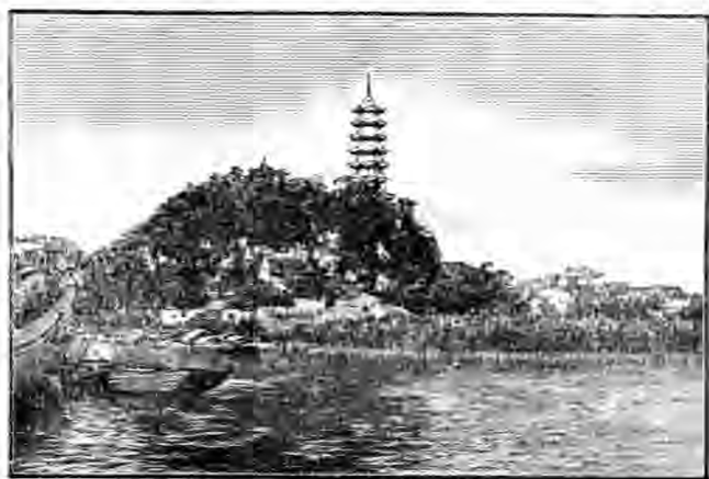
鎮江金山
