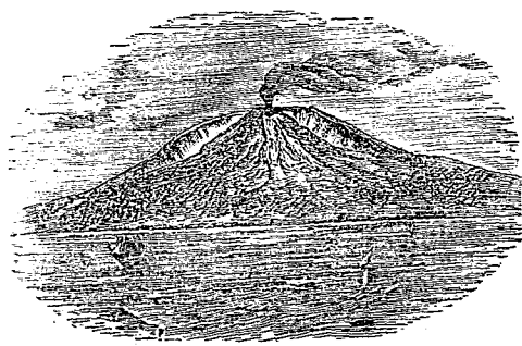
山 火
