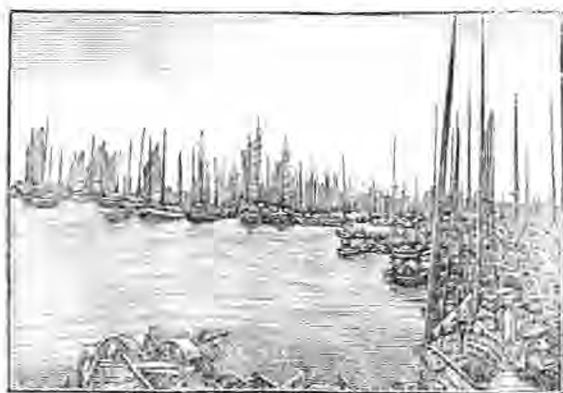
漢口
