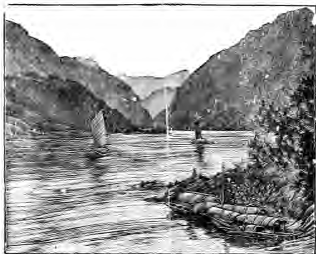
宜昌峽江
