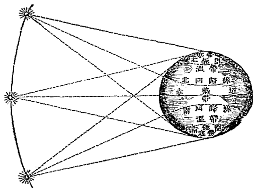
氣候帶五
