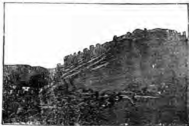
鎮南關
