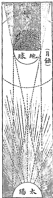
月蝕
