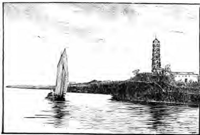
江 九
