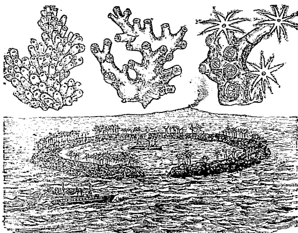
礁 環 瑚 珊
