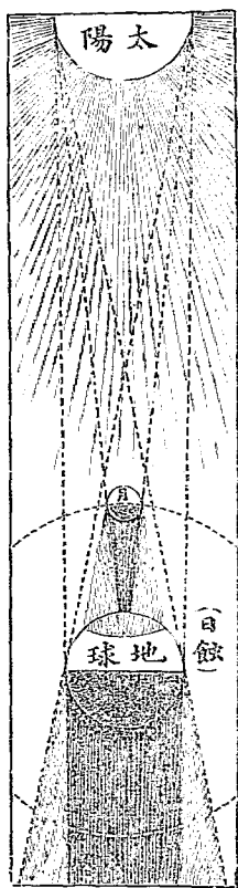
日蝕
