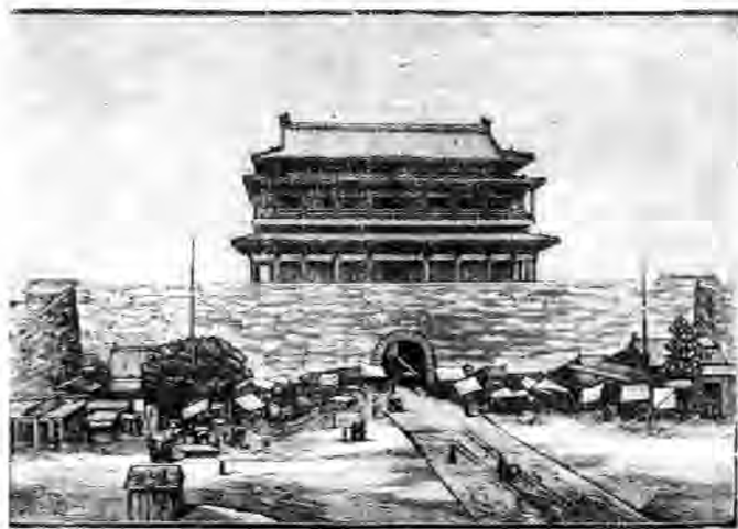
京師五陽門
