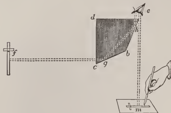
Camera Lucida.
