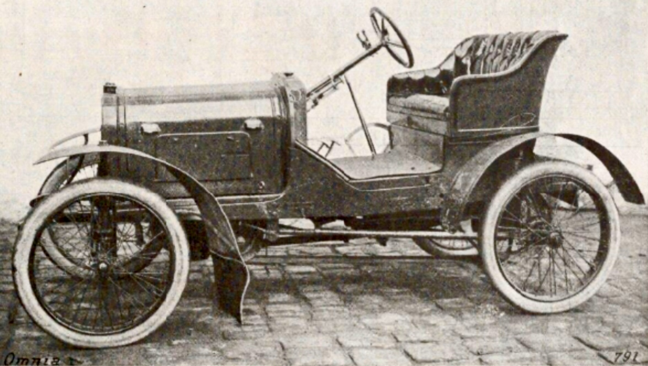
fig. 1. — La nouvelle voiturette Truffault.
