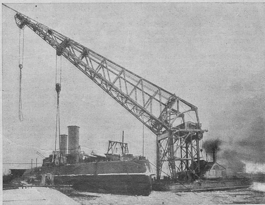
Новый двухсоттонный кранъ Балтійскаго завода.
