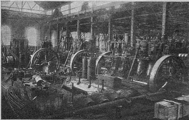
Сборочная Двигатель-моторовъ.
