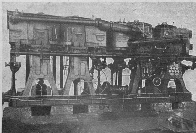
Одна изъ машинъ крейсера «Память Меркурія».
