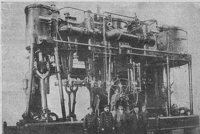
Одна изъ лучшихъ машинъ для броненосца «Іоаннъ Златоустъ».
