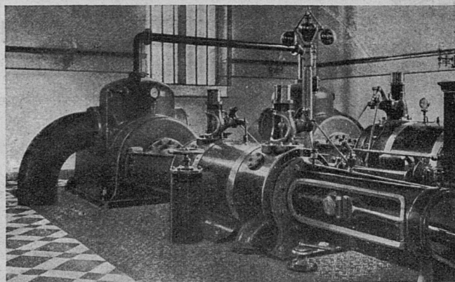
Паровая машина системы Ванъ-Денъ-Кернове.
