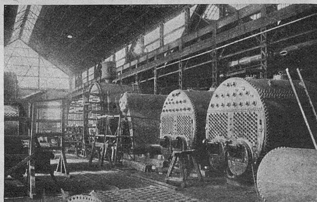
Котельная мастерская.
