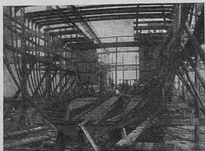
Постройка парохода «Малороссія».
