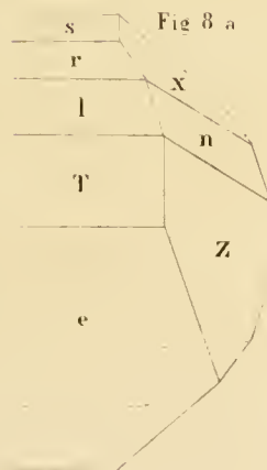
Fig. 1 & 2. Kristall af Ixiolit. Fig. 3. Dubbel kristall af Ixiolit. Fig. 4. Kristall af Tantalit. Fig. 5. Dubbel kristall af Tantalit. Fig. 6. Oregelvärdigt utbildad dubbel kristall af Tantalit (projektion emot basiska genomskärningen). Fig. 7. Genomskäring af en tvilling kristall af Tantalit. Fig. 8. Kristall af Orthit.
