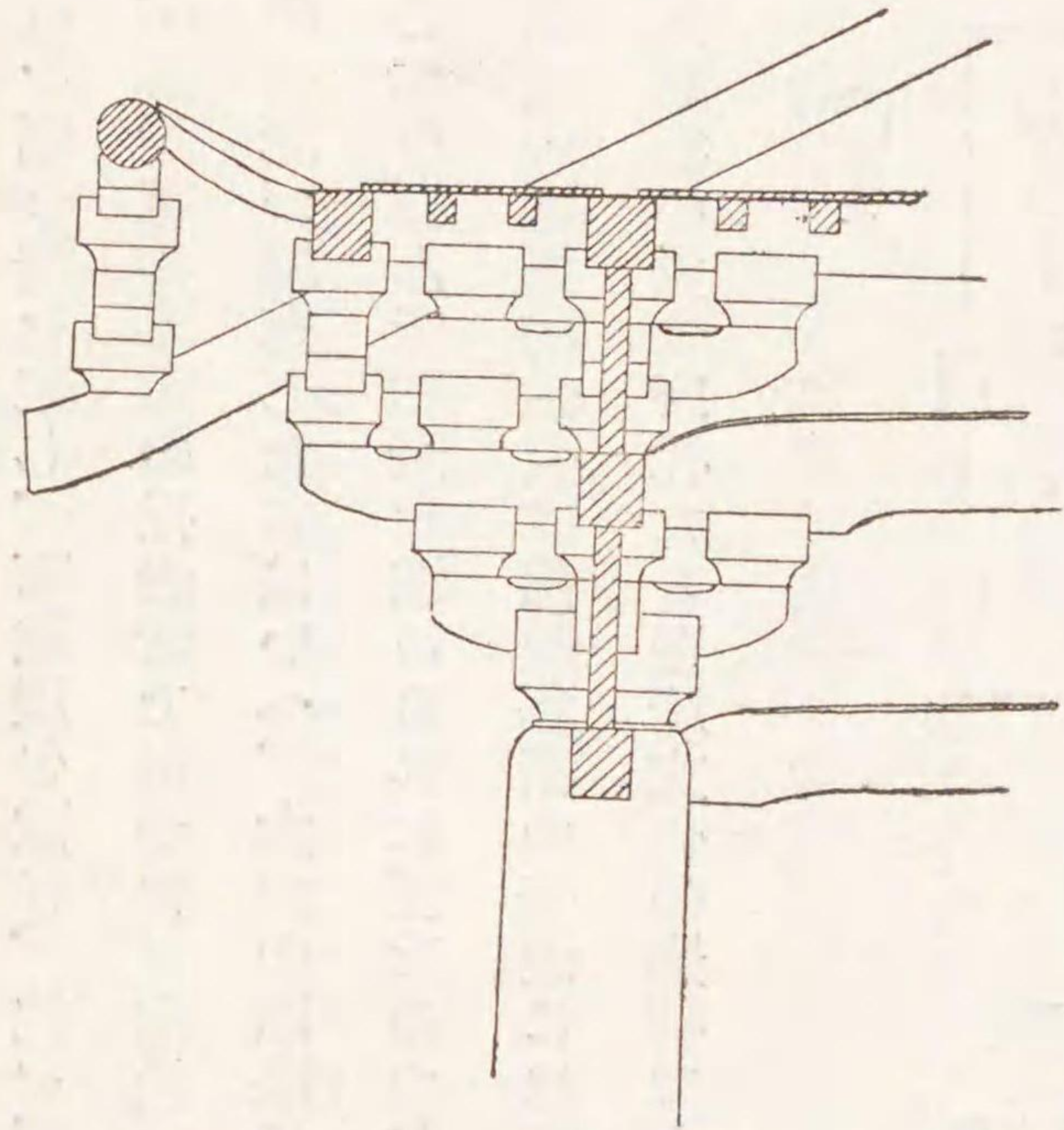
第十圖 三手先組物(唐招提寺金堂)
