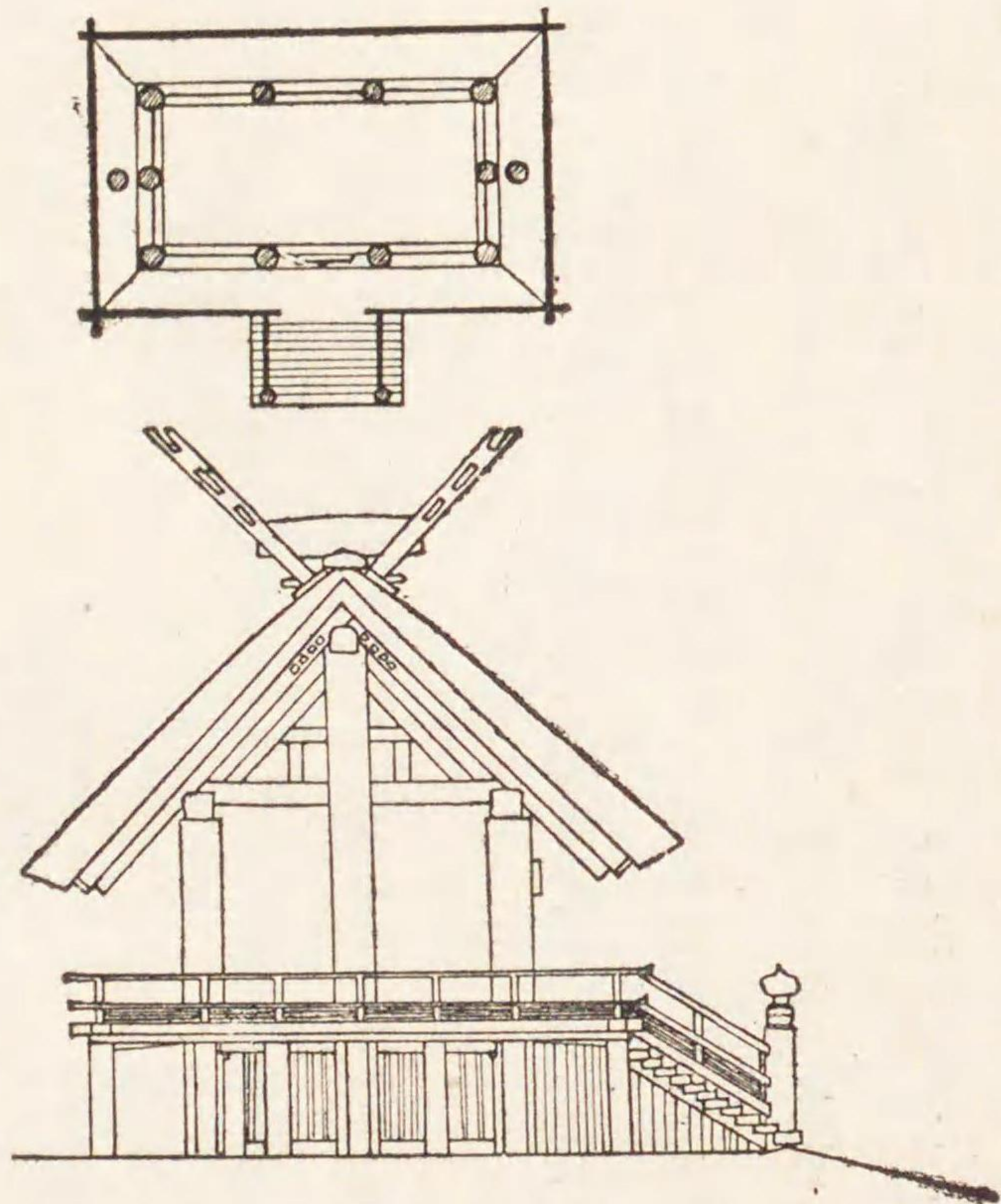
丙圖二第 伊勢神宮平面圖及側面圖
