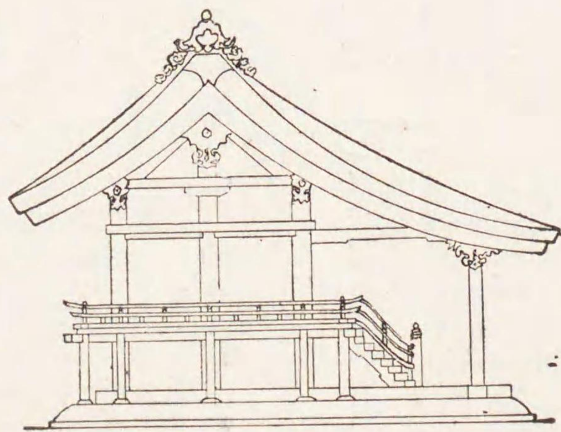
圖面側造流 乙圖三十第
