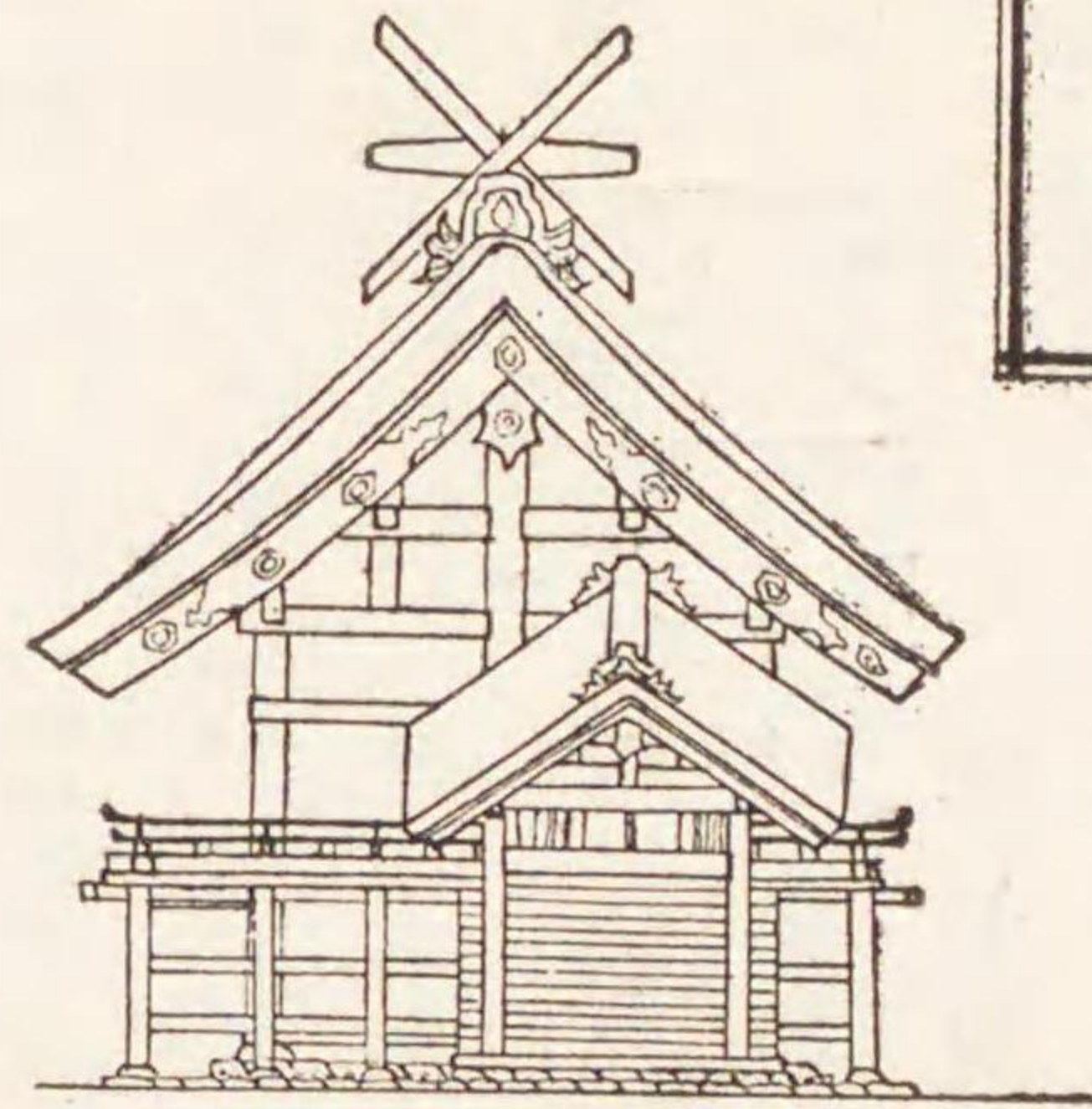
甲圖二第 出雲大神社平面圖及正面圖
