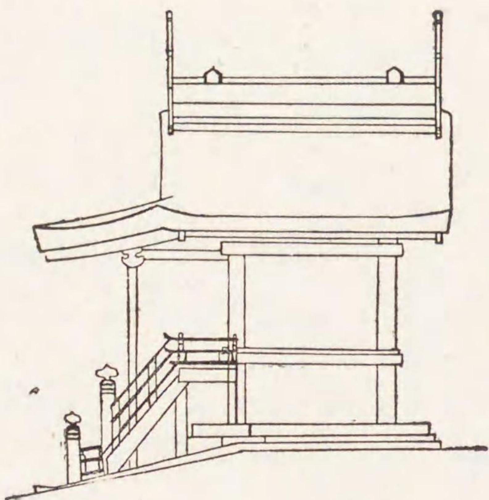
圖面側造日春 甲圖三十第
