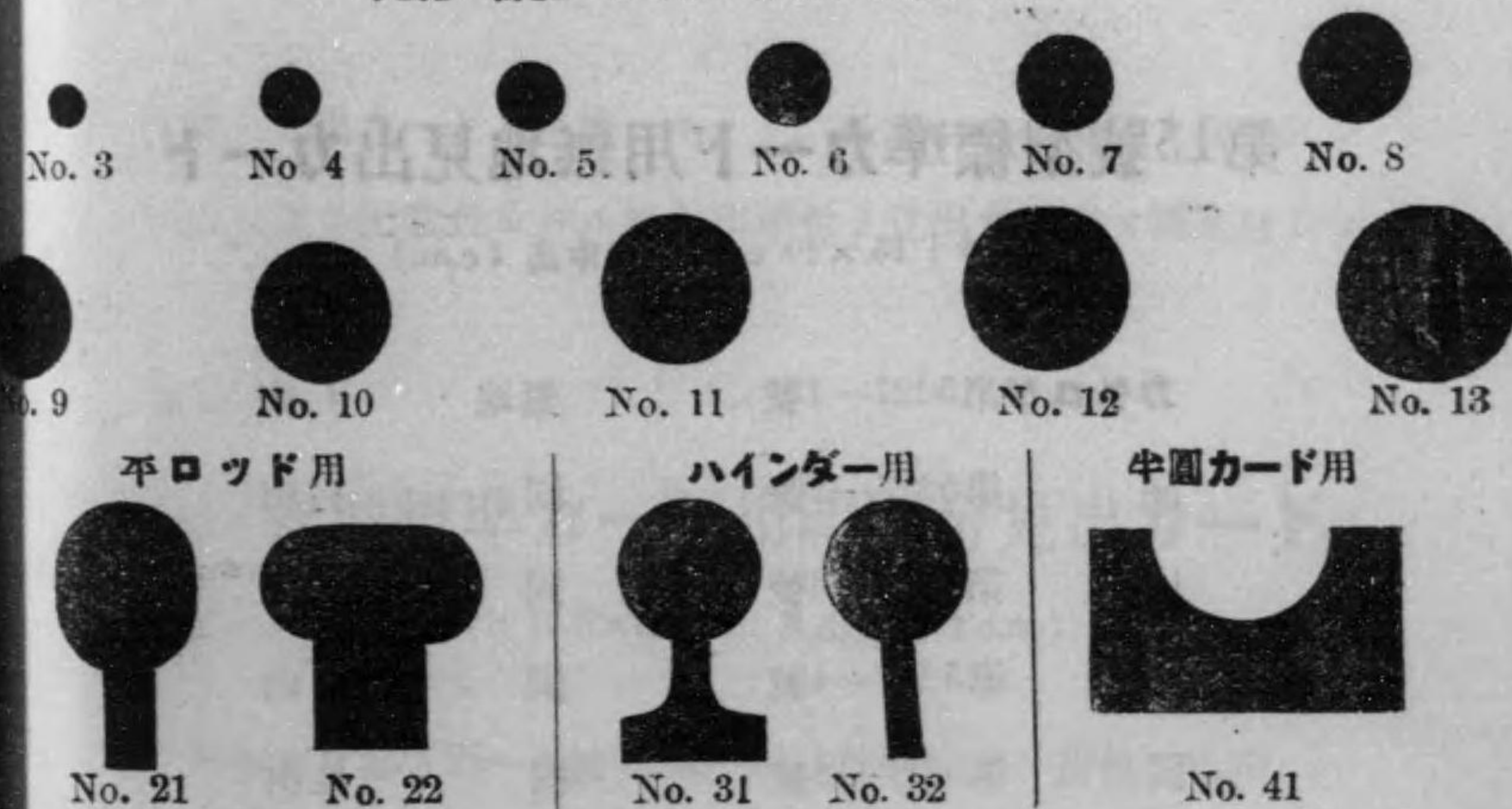
丸ロツド用丸孔 (丸孔ノ番號ハミリメートルテ直徑ヲ示ス)
