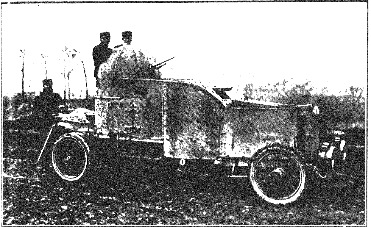
圖之射擊以上車汽甲裝於置砲關機用
