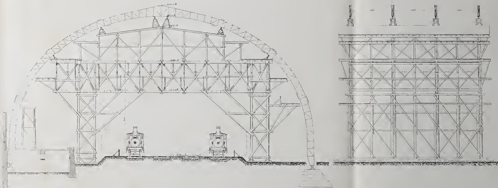
Voor-aanzicht
