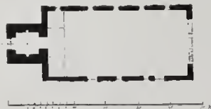
Grondplan
