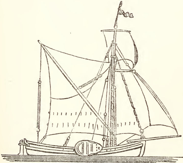
FIG. 26.—SAIL PLAN OF KOF-TJALK.
