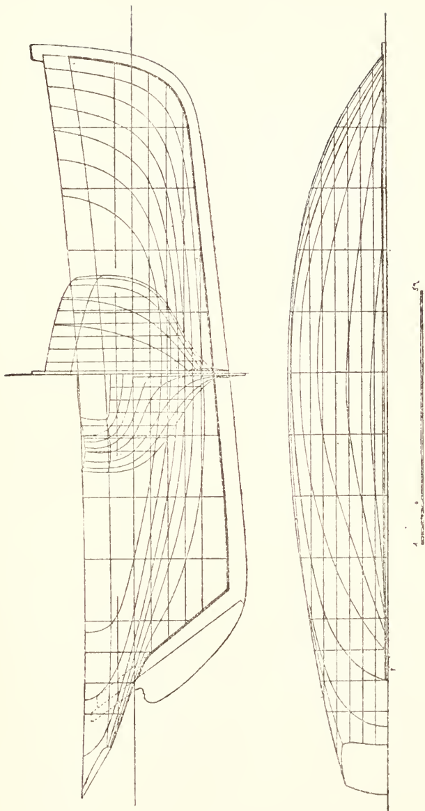
FIG. 117.—LINES OF ST. MALO CHASSE-MARÉE.
