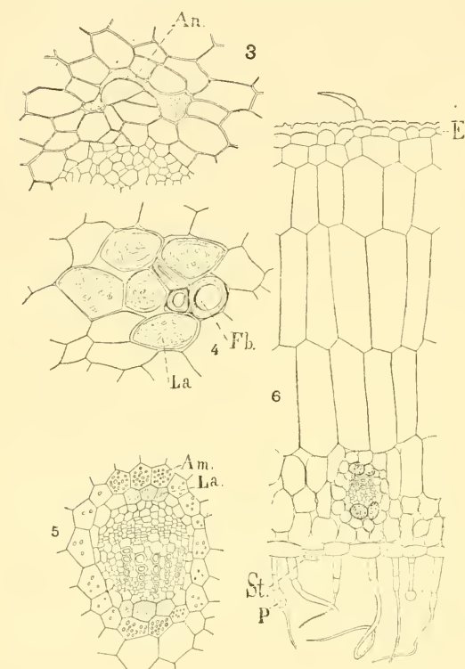
Fig. 3 à 6. — 3, région péryclicque de la souche rhizomateuse de Gazania splendens ; 4, même région dans la partie inférieure de la tige; 5, nervure principale vers l'extrémité de la feuille; 6, coupe transversale de la feuille. — Am , amidon; An , anastomose; E , épiderme; Fb , fibre; La , laticifères; P , poils; St , stomate.
