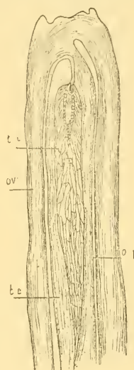
Fig. E — Ixida Helenium . — Mêmes lettres que précédemment.
