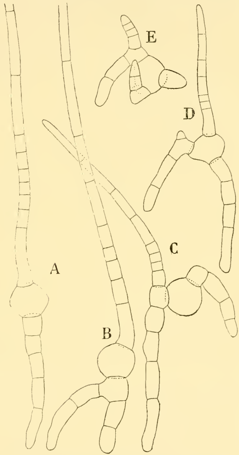
Fig. 3. — A. pusilla. — Propagules restés en culture du 19 au 30 avril. (Gross. 300.)
