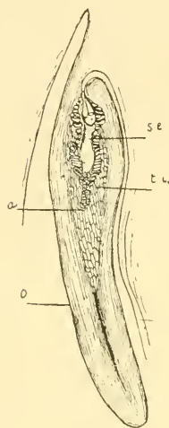
Fig. F. — Galatella rigida . — s. e., sac embryonnaire; a., antipodes; o., ovule; t. i., région interne du tégument.
