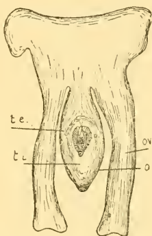
Fig. D. — Dahlia gracilis . — Mêmes lettres que précédemment.
