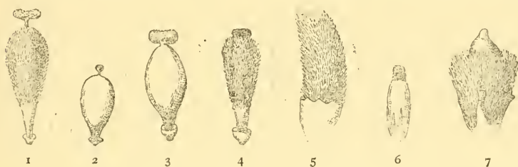
Fig. 1 à 7. — 1. Daphne Cneorum , ovaire. — 2. D. Laureola , id. — 3. D. Mezereum , id. — 4. D. Genkwa , id. — 5. Daphne composita , id. — 6. Wickstramia canescens , id. — 7. W. Balansæ , id.
