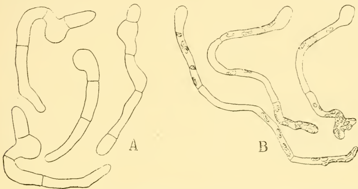
Fig. 1. — A. pusilla. — A, Germinations des zoospores des sporanges pluriloculaires; B, Germinations des zoospores des sporanges uniloculaires; A et B, sont de même âge, du 10 au 13 avril. (Gross. 300.)
