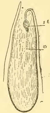
Fig. J. — Echinacea intermedia.
