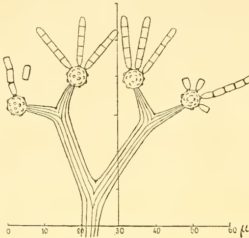
Fig. 6. — Piptocephalis sphærocephala , n. sp.
