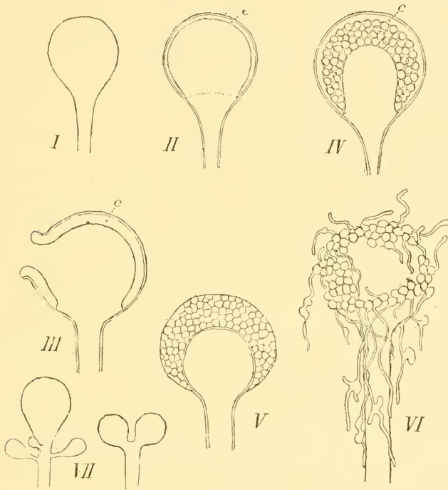
Fig. 1. — I-IV. Développement de la membrane du sporange de Rhizopus nigricans . I° Sporangium jeune à membrane homogène; II, sporangium dont toute la paroi interne s'est doublée d'un revêtement de callose c ; III, le même sporangium traité par l'acide phosphorique qui a gonflé la couche de callose; IV, sporangium un peu avant la formation des spicules et montrant la couche de callose c moulée sur les spores en voie de formation.
