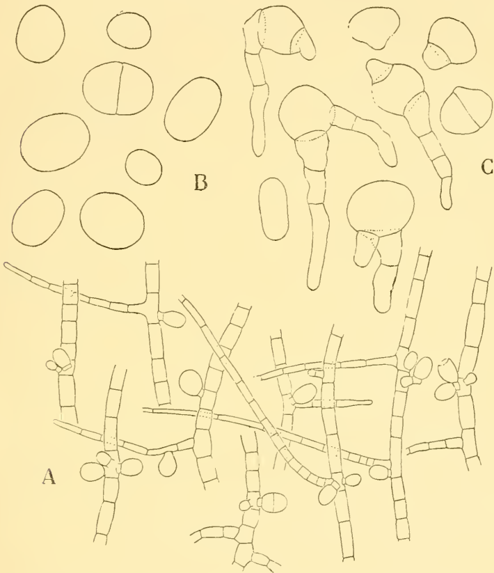
Fig. 2. — A. pusilla. — A, Fragments de filaments pour montrer la position des pseudo-sporanges. (Gross. 80.) — B, Propagules mûrs et fraîchement sortis, dessinés pour montrer leurs variations de forme et de dimensions. — C, Propagules restés en culture du 19 au 25 avril. (B et C. Gross. 200.)
