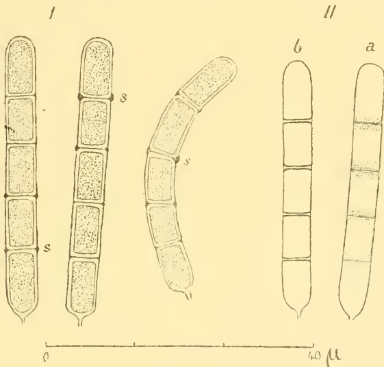
Fig. 2. — Sporangies de Piptocephalis arrhiza examinés avant la maturité. — A gauche, trois sporangies traités par l'alcool et colorés par les réactifs du protoplasme; les cloisons et la membrane externe sont incolores et l'on aperçoit sur les côtés, marquées en noir, des saillies formées par une substance mucilagineuse inerte vis-à-vis des réactifs colorants. — A droite, deux sporangies dépourvus de leur contenu et colorés par la benzoazurine; en a , les cloisons sont encore simples, en b elles sont dédoublées.
