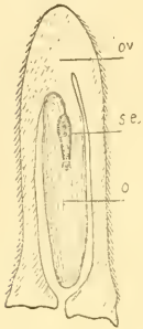
Fig. O. — Aster Novæ Angliæ . — Mêmes lettres que précédemment.
