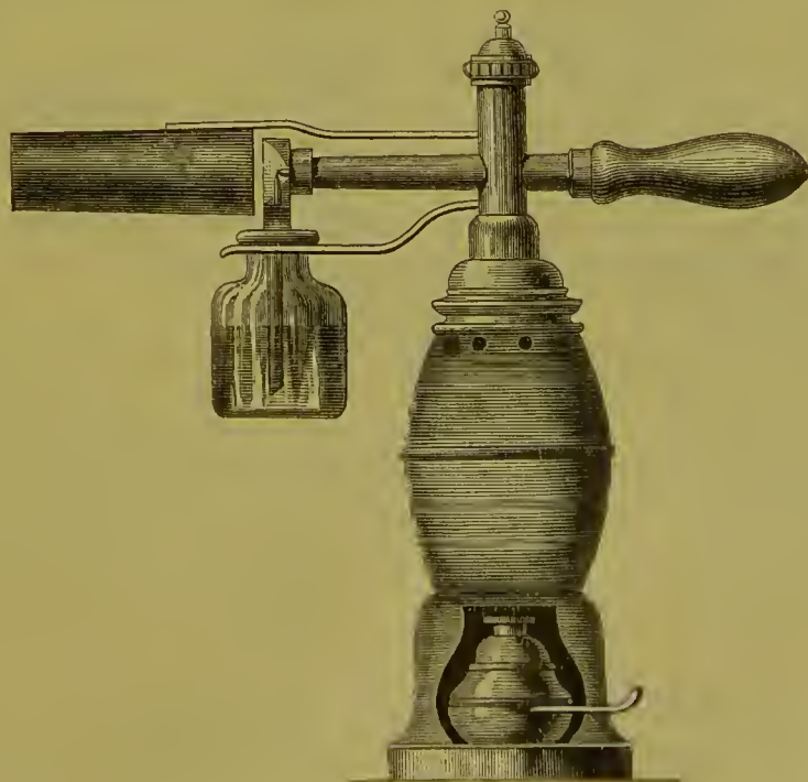
Apparat von Siegle.
