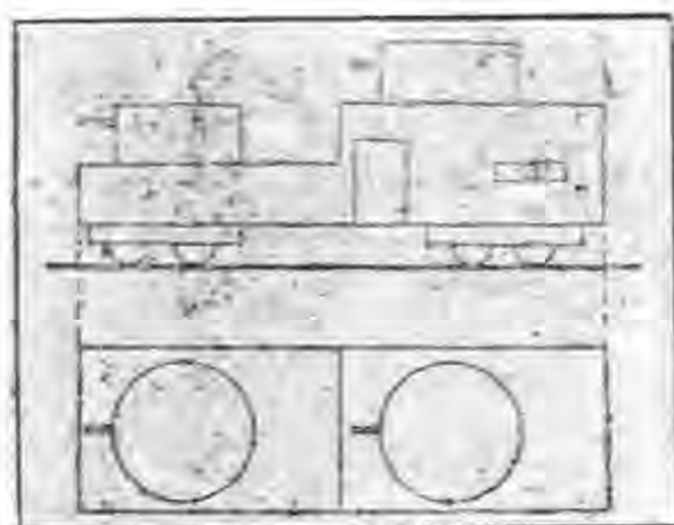
第 三 印 大 那 休 爾 號 火 砲 車 之 要 領 圖 第 三 圖
