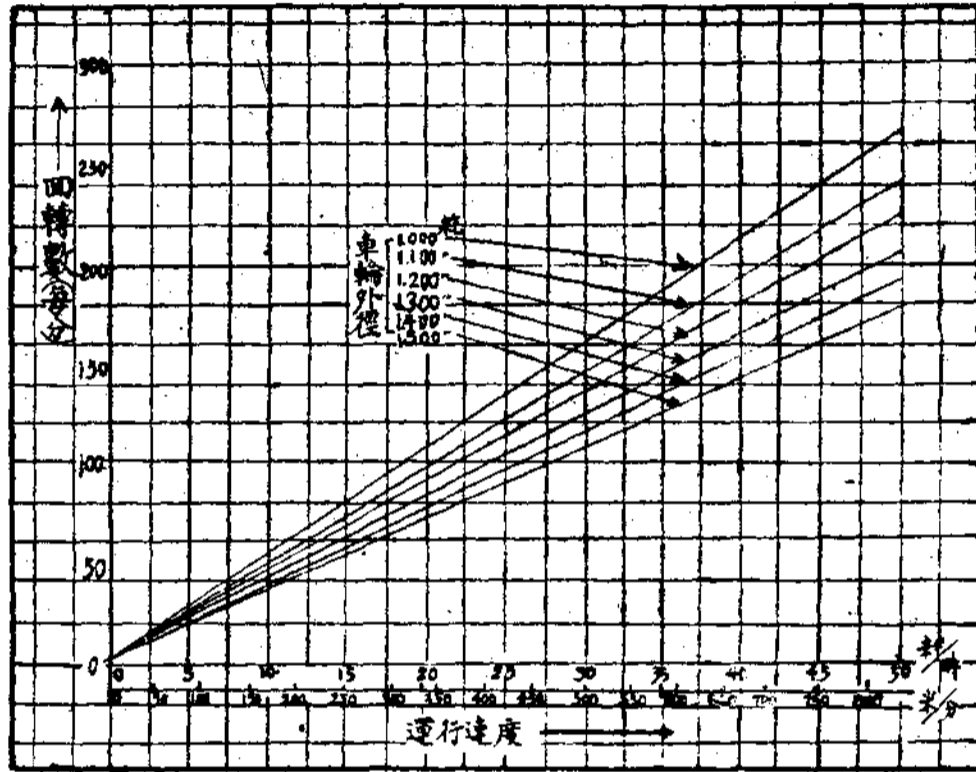
附圖 第一 火礮車輪運行速度與回轉數之關係
