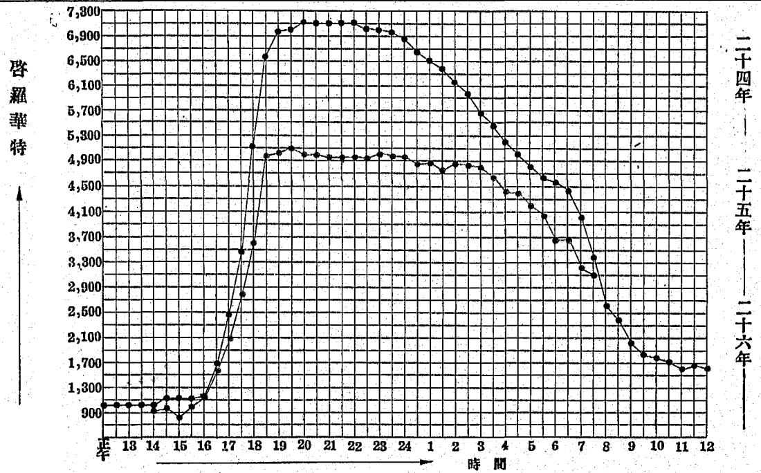
湖南電鑛公司發電廠民國二十四年二十五年二十六年舊歷除夕機械負荷比較圖
