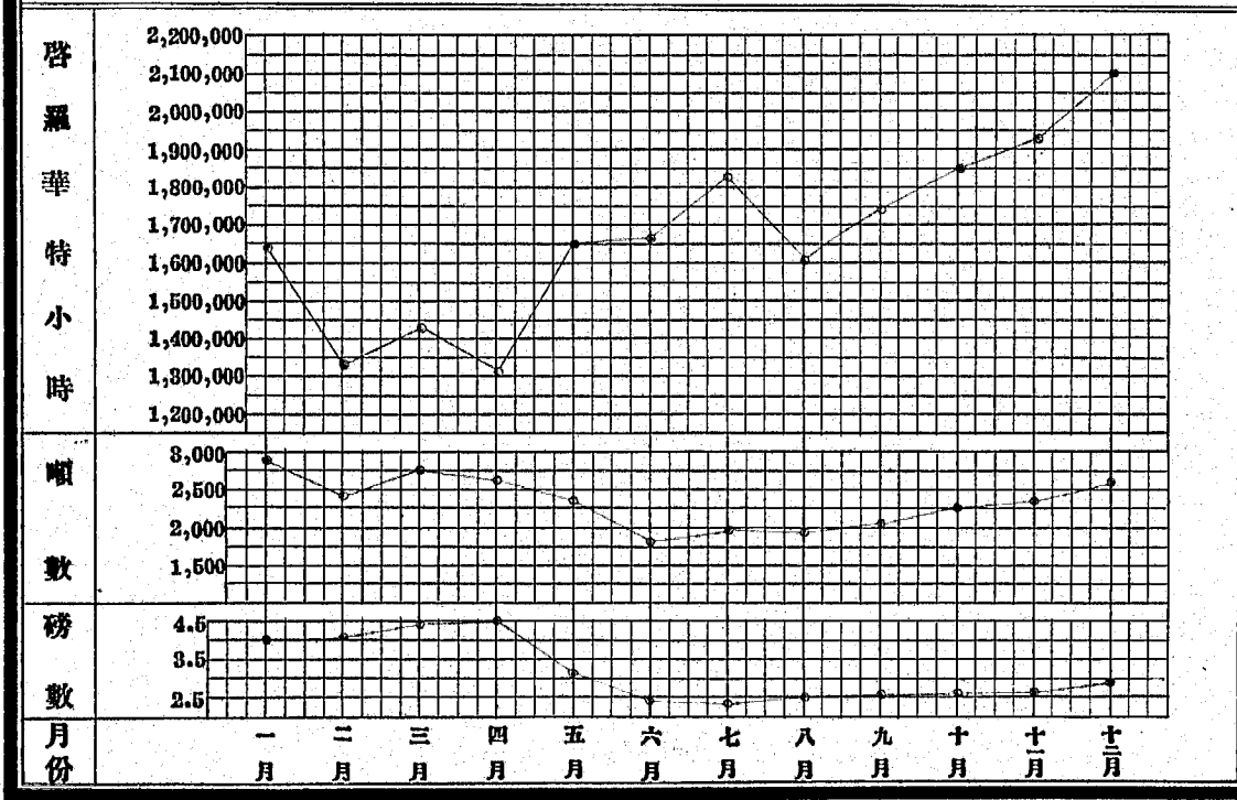
民國二十六年湖南電燈公司發電廠發電與燒煤逐月比較圖
