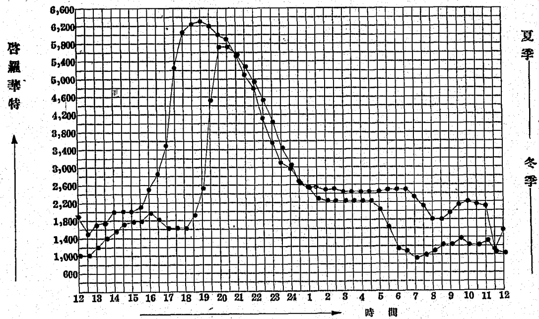
民國二十六年湖南電燈公司發電廠電機多夏負荷比較圖
