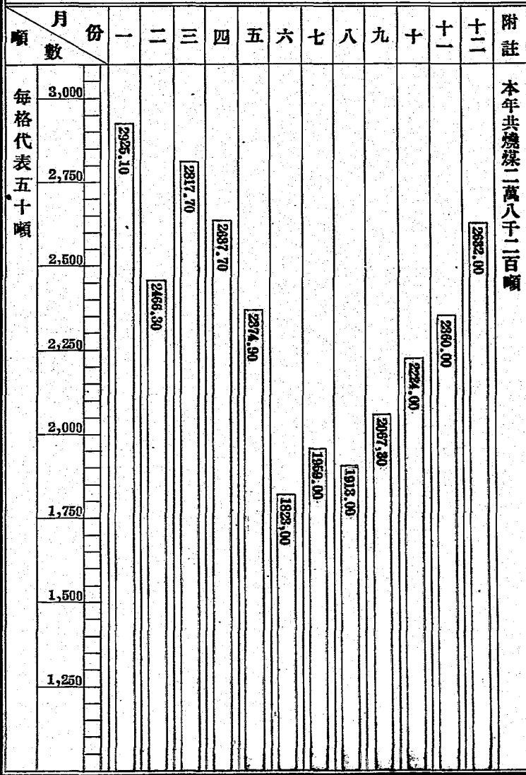
民國二十六年湖南電燈公司發電廠燒煤逐月比較圖
