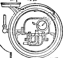
汽鍋水平切面圖
