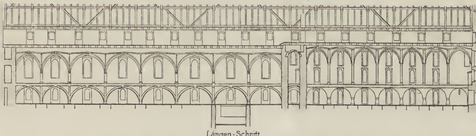
Längen-Schnitt
