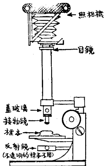
照相時的裝置法
