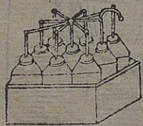
六 同上 數瓶 相連
