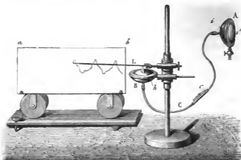
FIG. 38. — Cardiographe applicable à l'homme.
