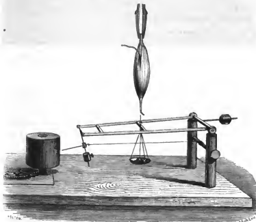
FIG. 135. — Myographe de Helmholtz.
