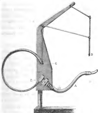
FIG. 44. — Kymographion à ressort de Fick.
