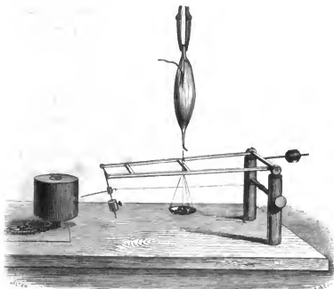
FIG. 28. — Myographe de Helmholtz.
