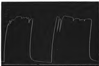
FIG. 127. — Deux périodes du téтанos provoquées par un courant constant appliqué au nerf.
