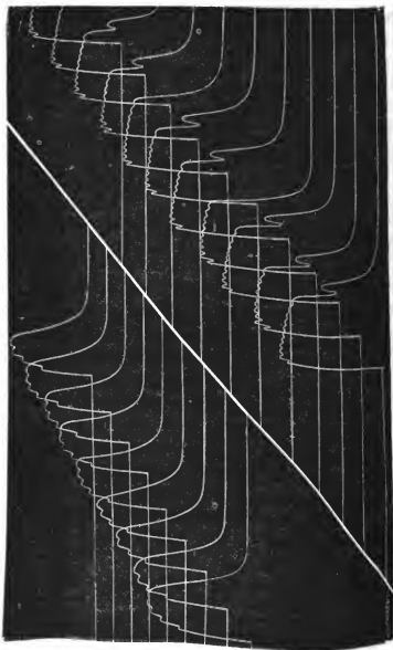
Fig. 132. — Deux séries d'accès tétoniques disposées en l'embrasure oblique. — Le grenouille est empoussinée depuis vingt-quatre heures. — La série inférieure est obtenue la première. — La supérieure est enregistrée après cinquante minutes d'excitations répétées à chaque minute.
