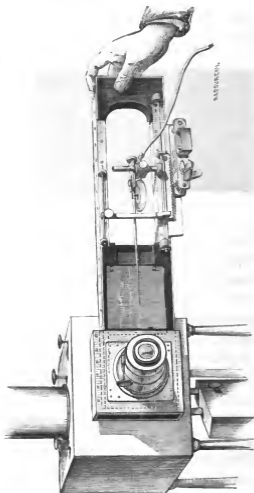
Fig. 55. — Polygraphe à projection. — L'appareil est représenté au moment où un le retire du mégascope à lumière électrique dans lequel il a tracé des graphiques de mouvements qui lui étaient transmis à une distance de 45 mètres au moyen d'un tube de caoutchouc. On voyait les graphiques se former en traits lumineux sur l'écran. Ces figures étaient amplifiées environ à 30 diamètres.
