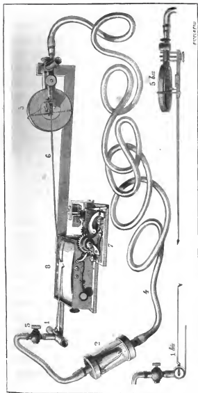
FIG. 47. — Hémigraphie de Chauveau et sphygmographe enregistrant simultanément leurs indications.
