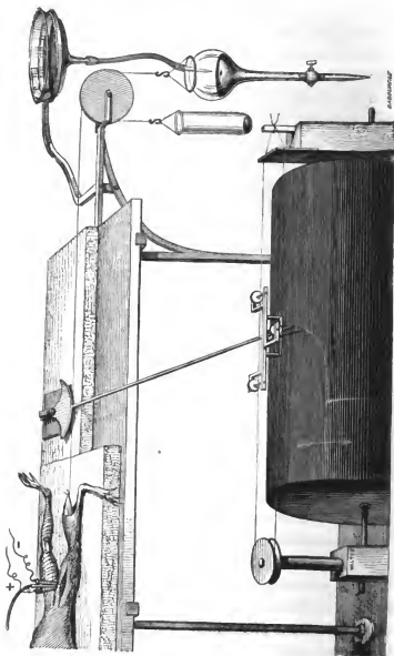
Fig. 91. — Appareil enregistreur de l'élasticité des corps.
