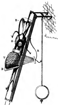
FIG. 5. — Schéma du choc du cœur.
