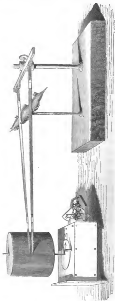
FIG. 84. — Deux leviers simples disposés pour enregistrer le passage de l'onde musculaire.
