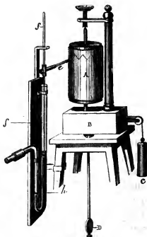
FIG. 27. — Kymographion de Ludwig.
