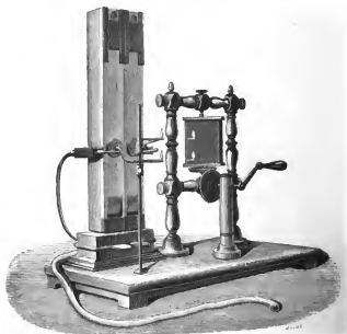
FIG. 20. — Appareil de M. Kœnig servant à l'analyse des sons par la méthode des flammes manométriques.
