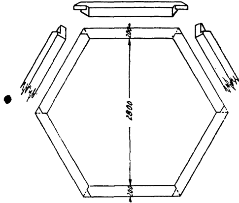
六角蓋
