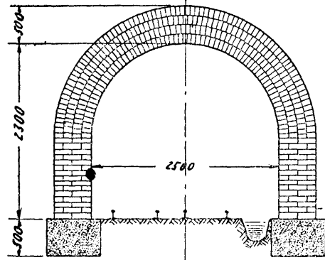
磚 圈
