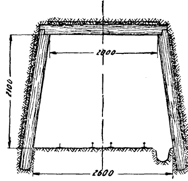
木架
