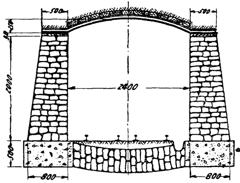
鐵梁塊石棚
