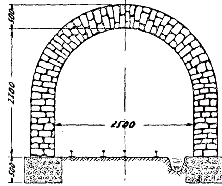
塊石圈
