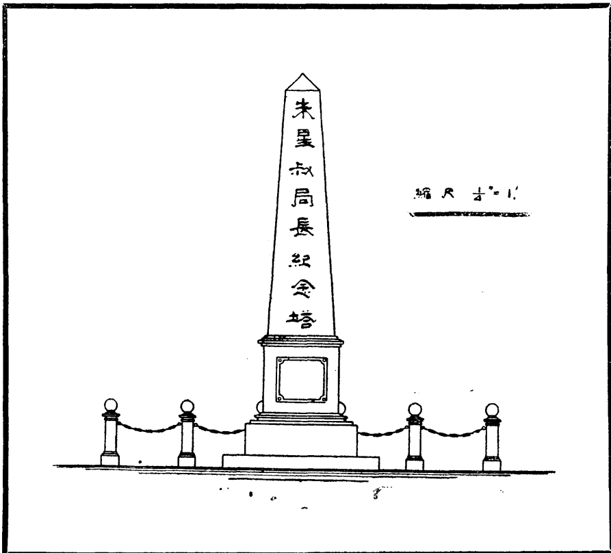
乙 紀念塔設計圖
