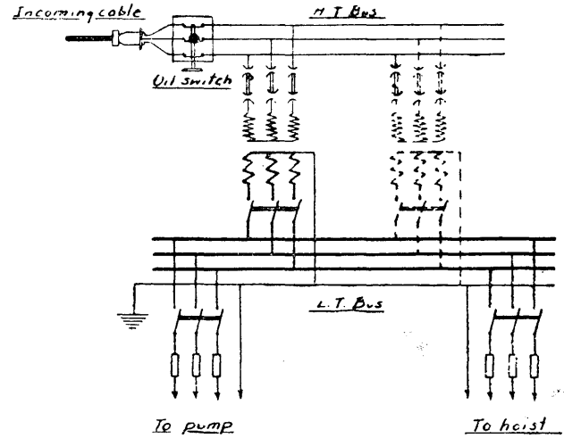
建設委員會與煤礦局 四機井井下變壓所圖 民國二十年六月建造 縮尺 1:1
