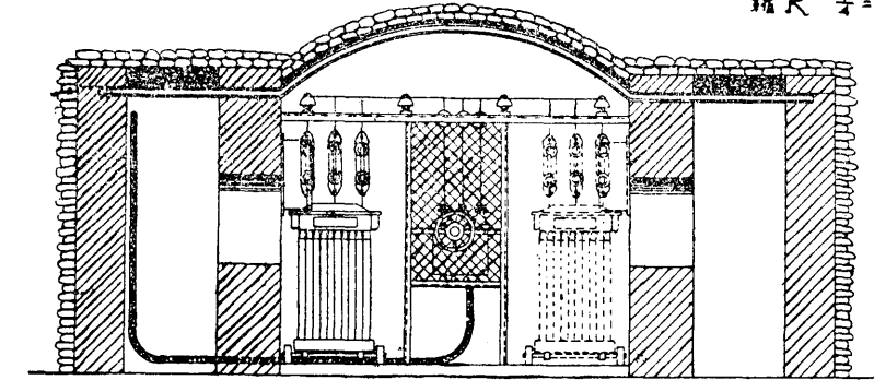
建設委員會與煤礦局 四機井井下變壓所圖 民國二十年六月建造 縮尺 1:1
