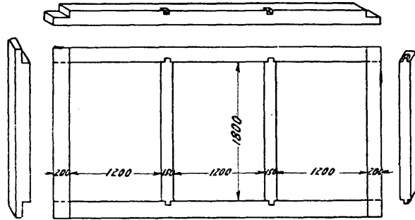
四方蓋
