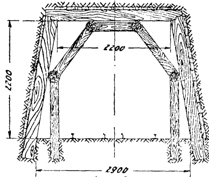
木 架
