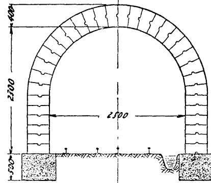
洋灰磚圈
