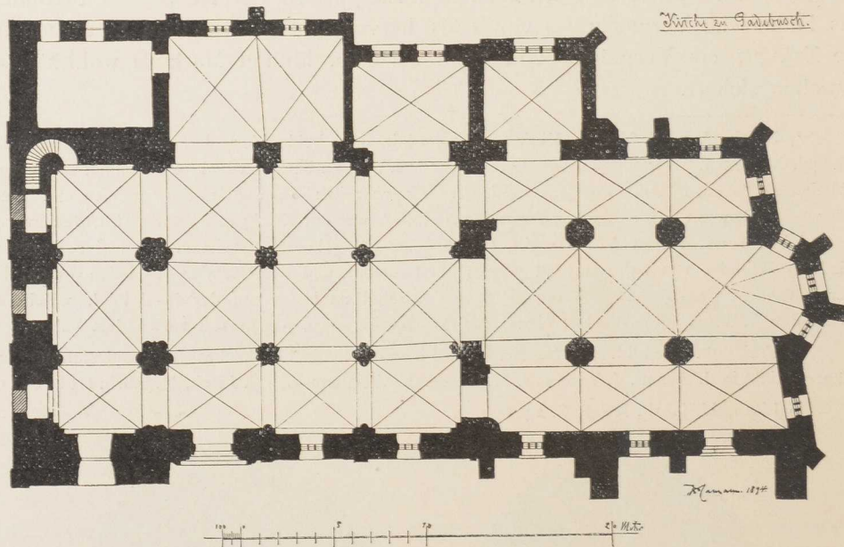
Grundriss der Kirche zu Gadebusch. Nach Hamann.
