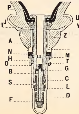
COUPE DE LA VALVE VOITURE Modèle 1903
