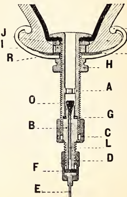
COUPE DE LA VALVE "TERMINUS" Modèle 1898
