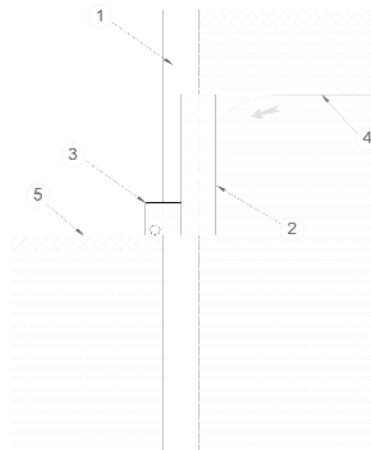
Fig. 21 Incinta drenanta 1-Perete perimetral din piloți forati cu interspații; 2- Dren vertical între pilotii forati pentru colectarea apelor freatice; 3-Dren longitudinal; 4-Nivelul apei freatice care curg spre incinta; 5-Teren existent; 6-Limita inferioara a excavatiei
