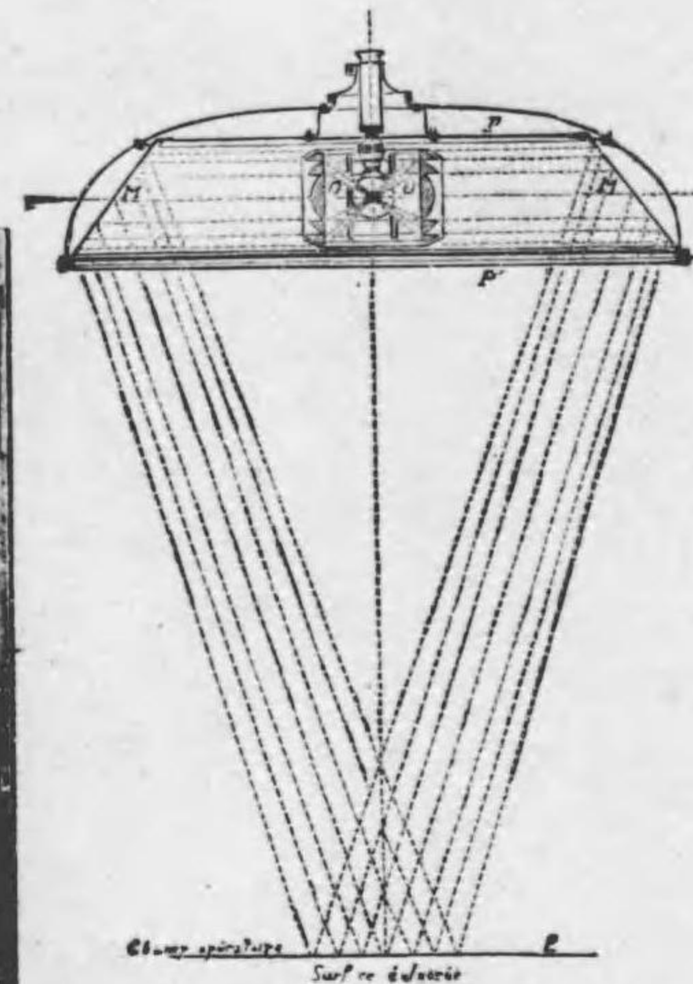
Q 240-244 無影照明ノ原理ヲ示セル圖
