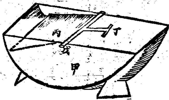
花生剝殼機
