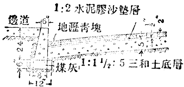
第六十二圖 地瀝青塊路橫剖面
