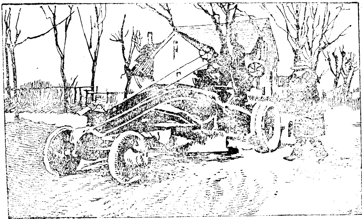
第三十四圖 削路機汽車
