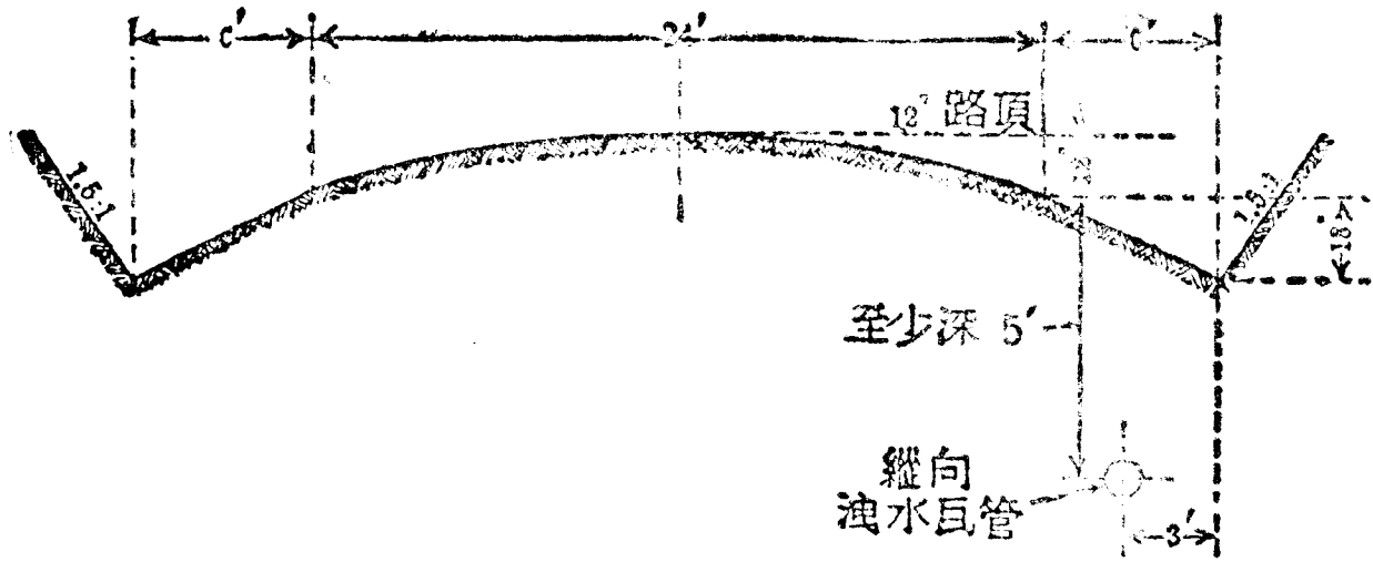
第二十四圖 坡度在百分之二至百分之四之間之 土路橫剖面
