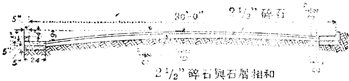
第五十六圖 瀝青碎石路橫剖面
