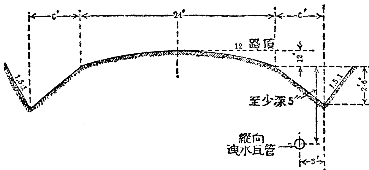
第二十三圖 坡度在百分之二以下之土路橫剖面
