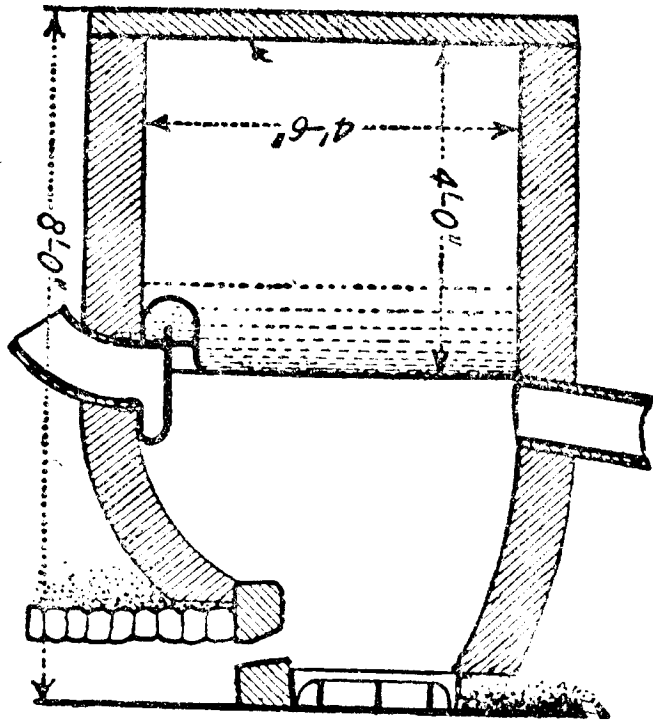
第七十一圖 人行路下之集水塘
