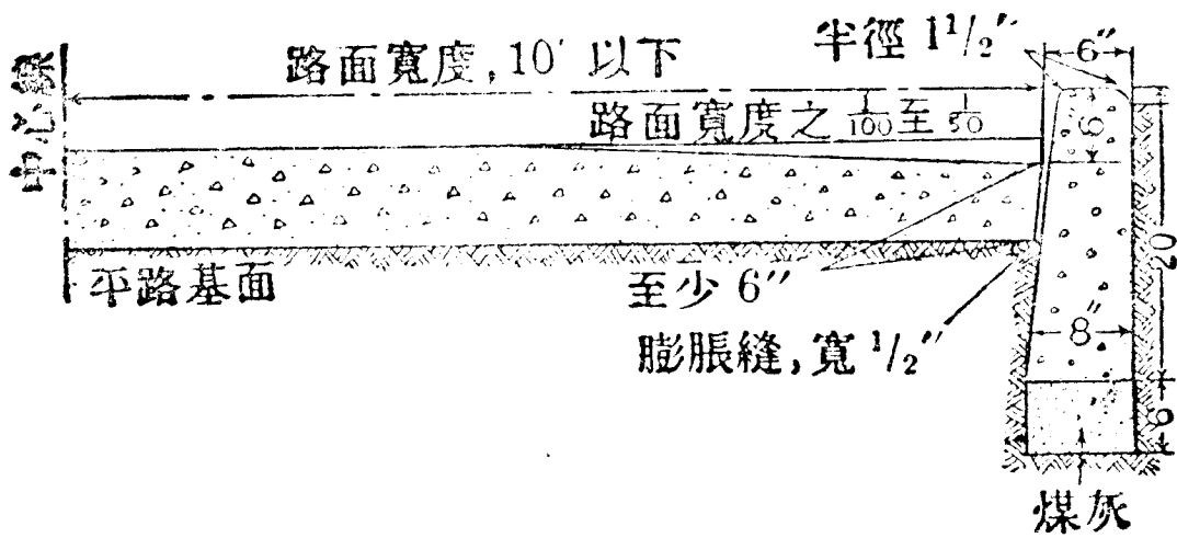
(甲)無鋼骨三和土
