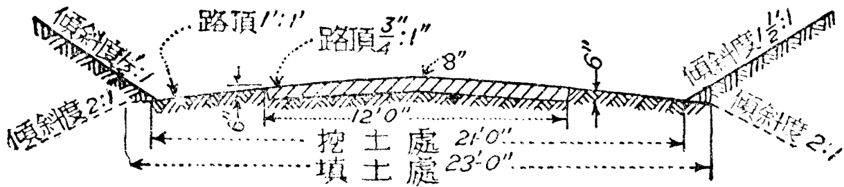
第三十三圖 卵石路橫剖面
