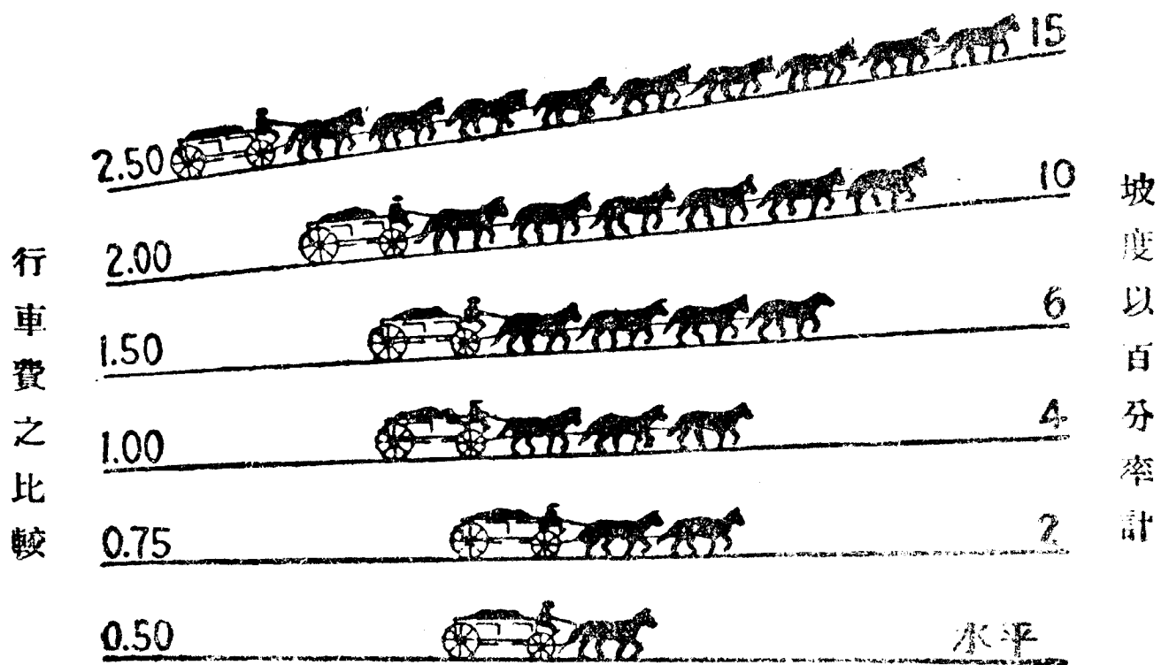
第三圖 斜坡對於行車力之影響
