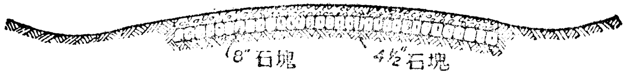
第三十五圖 威爾福德式碎石路橫剖面
