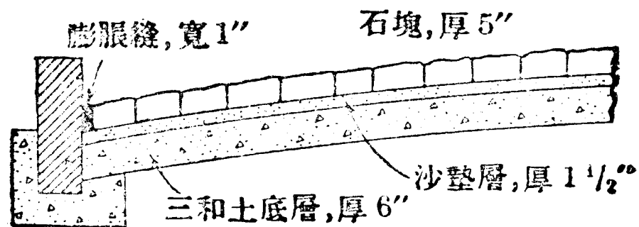
第四十五圖 花崗石塊路橫剖面
