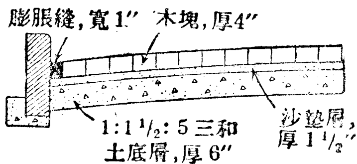
第五十二圖 木塊路橫剖面
