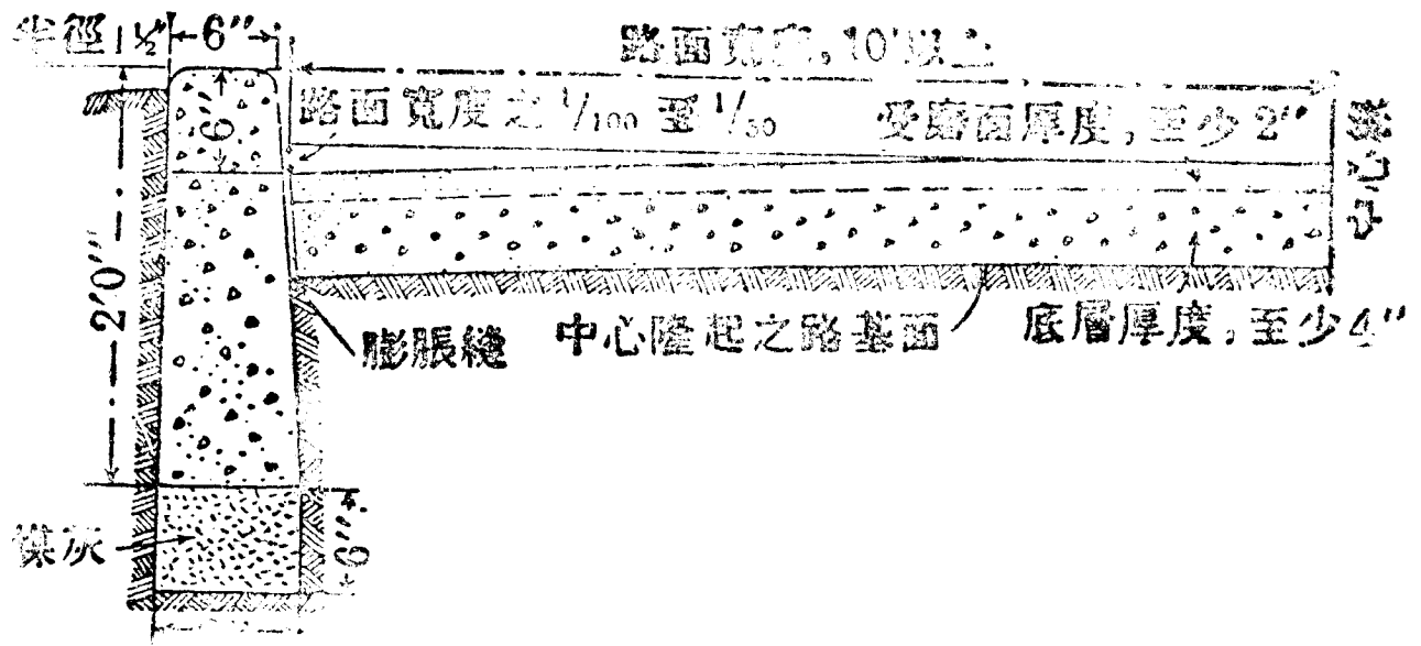
第四十一圖 二層式三和土城市道路橫剖面
