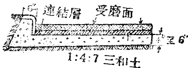
第五十九圖 地瀝青片路橫剖面
