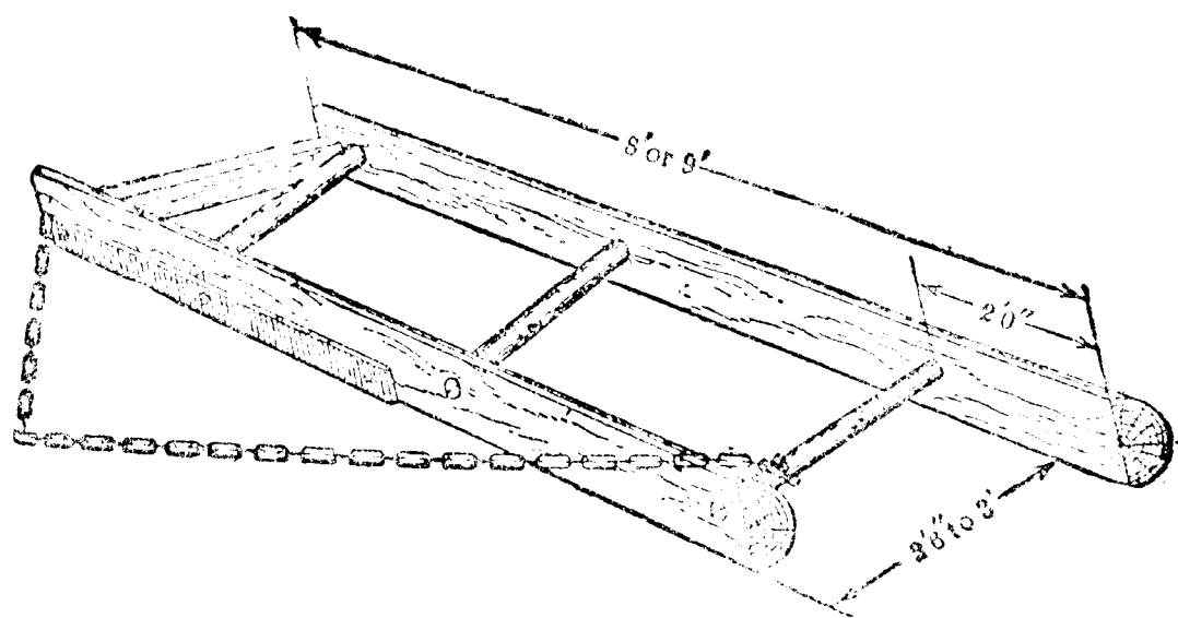
第二十八圖 馬曳對劈圓木刮路器
