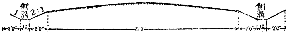
第六十七圖 斜岸平底側溝
