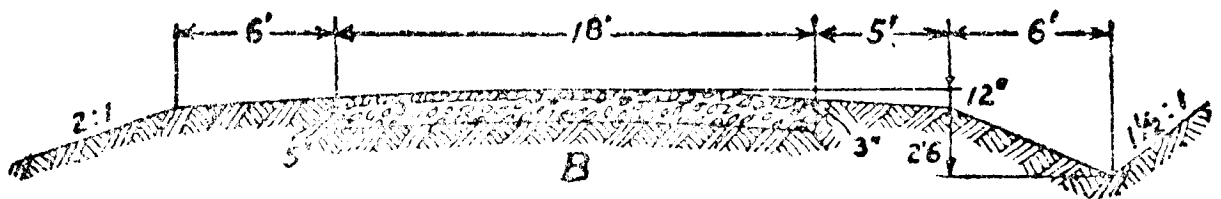
第三十六圖 馬卡丹式碎石路橫剖面
