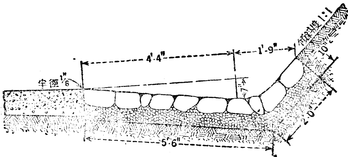
第六十八圖 石側溝
