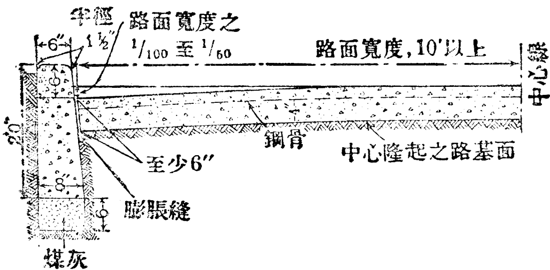
(乙)鋼骨三和土
