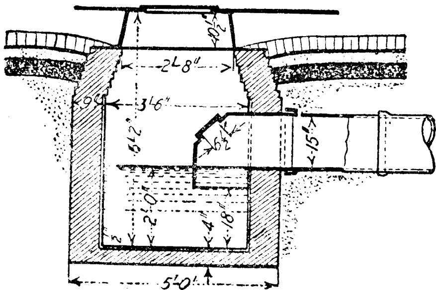
第七十二圖 側溝下之集水塘
