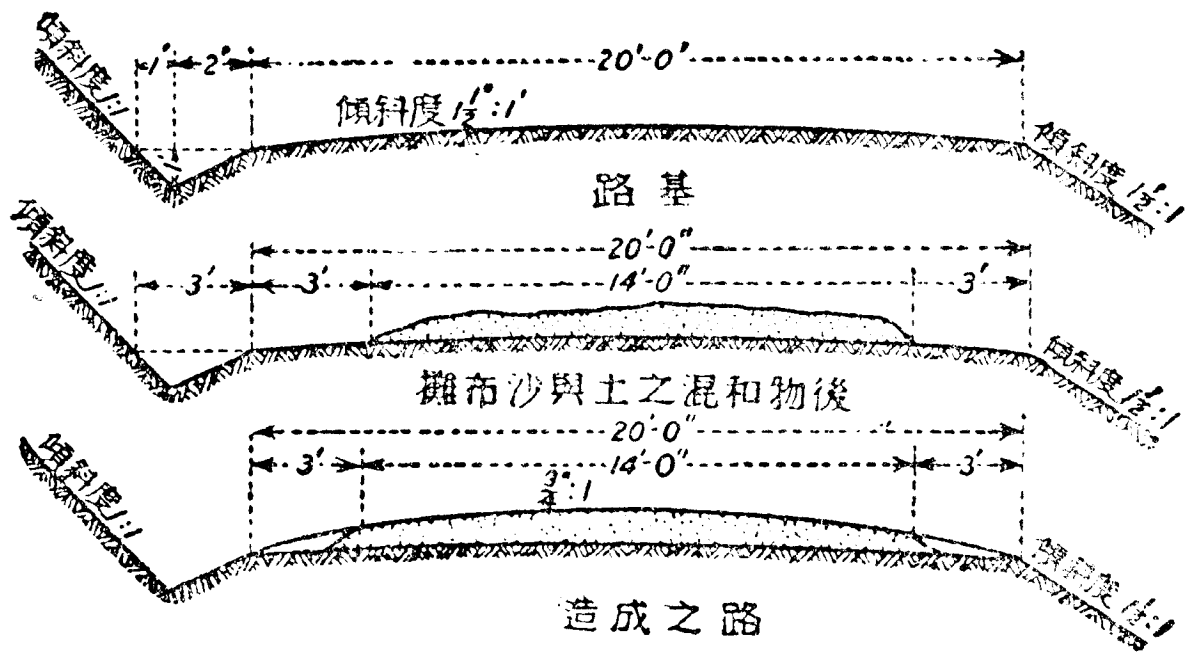
第三十一圖 沙土路之築造程序
