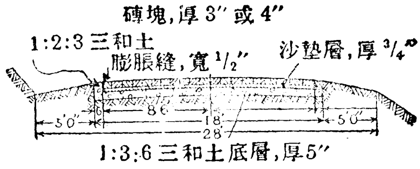
第四十八圖 磚路橫剖面
