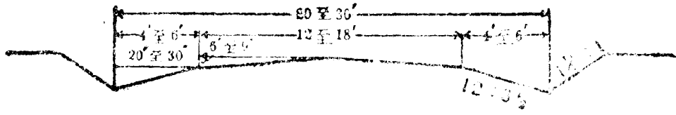
第六十五圖 尖底側溝
