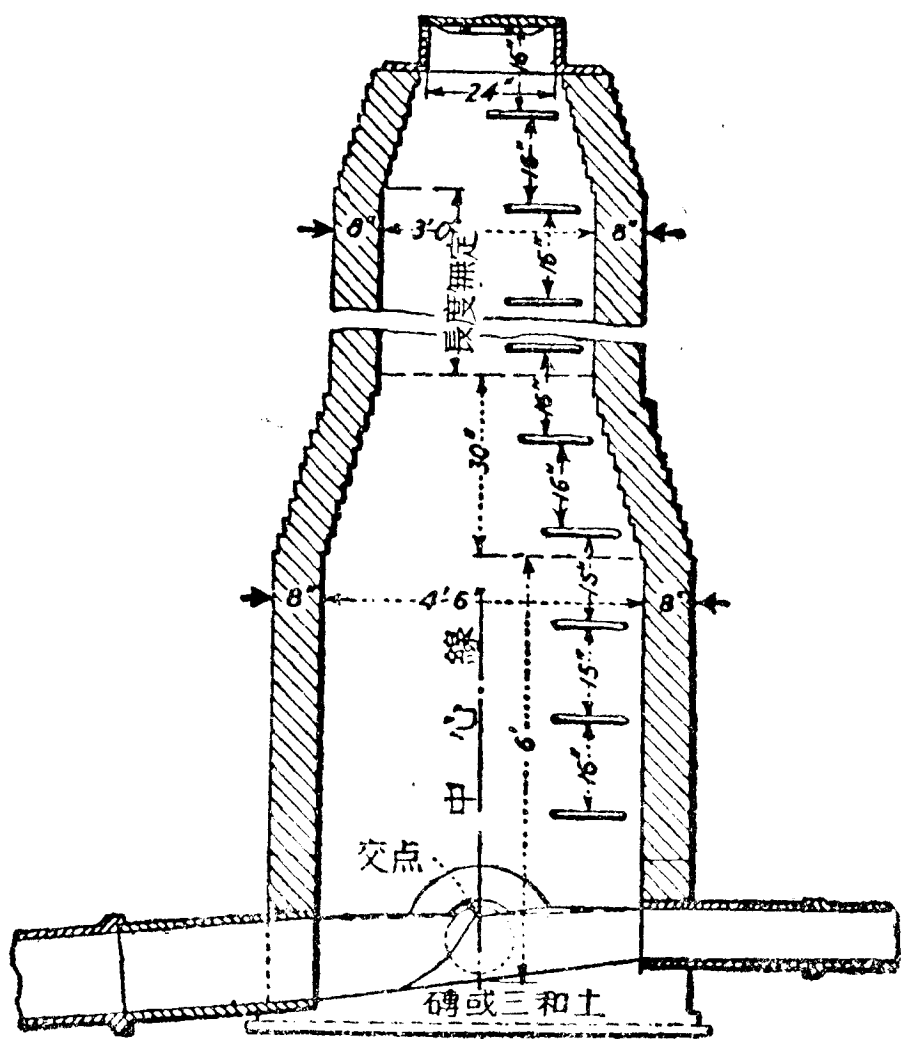
第七十三圖 人井
