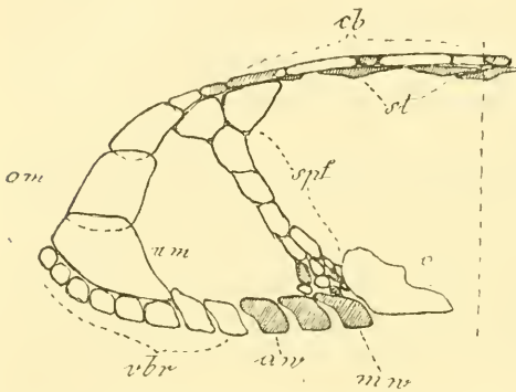
Fig. 3. Schematisirter Interradialerschnitt durch das Skelett von Culcita schmideliana Retz. cb. Dorsale Connectivbalken; st. Sternplatten; om. Obere Marginalplatte; um. Untere Marginalplatte; vbr. Ventrale Brachialia; aw. Armwinkelplatte, mw. Mundwinkelplatte; o. Orale; spf. Septalpfiler.
