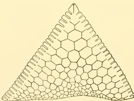
Fig. 1. Ventralskelett von Calcita schmidliana Retz. nach Viguier l. c.
