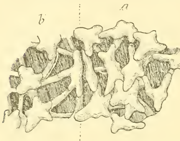
Fig. 4. Stück aus dem dorsalen Skelett von Calcuta schmideliana Retz. von der Unterseite. a. Centrale Region; b. Periphere Region.
