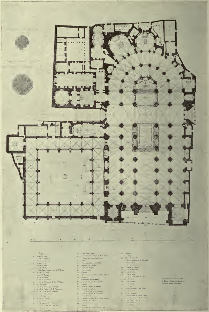
PLAN OF THE SANTA IGLESIA PRIMADA
