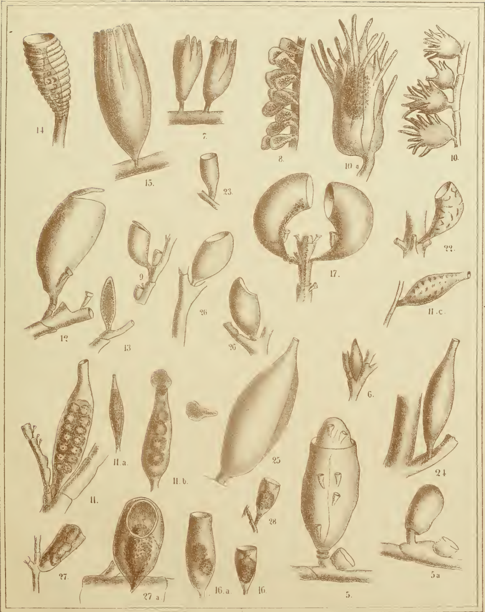
Gonotheken: 5-17. Plumularia; 19-27. Nemertesia.
