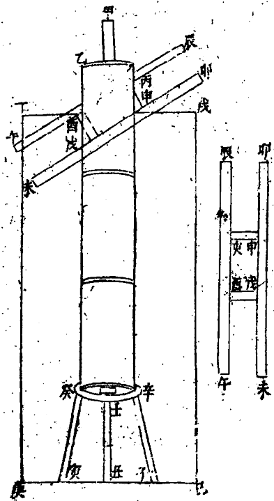
恒升四圖
