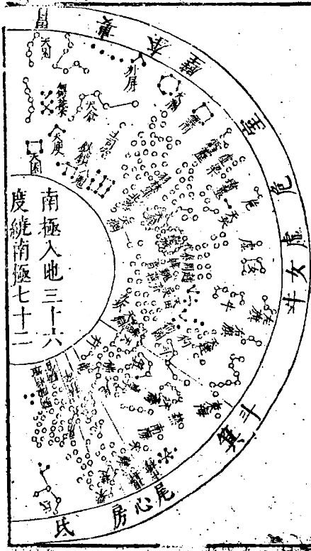
渾天南極圖
