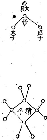
心宿圖
