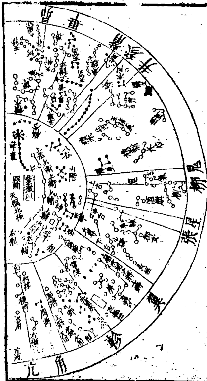
渾天北極圖
