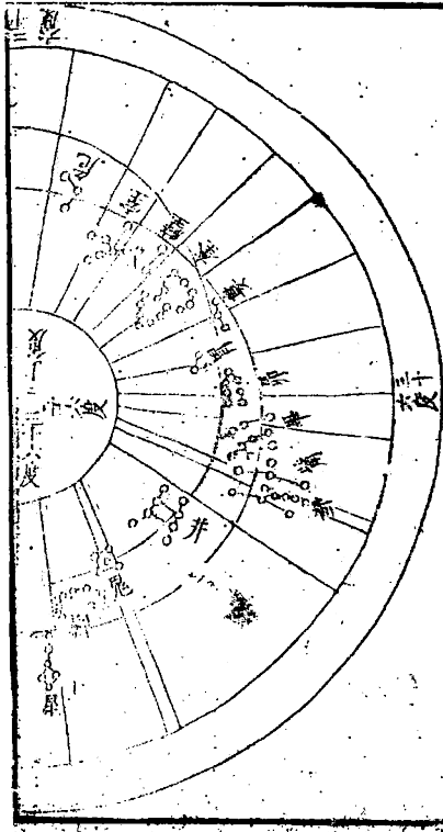
蓋天圖
