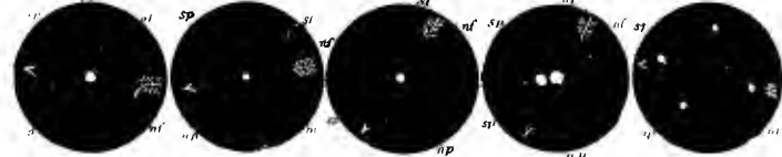
ζ Orionis η Monocerotis ε Hydræ Castor Trapezium
