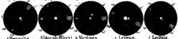
ζ Herculis Algorab (δ Corvi) γ Virginis γ Leonis ι Leonis
