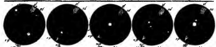
ζ Lyrae η Lyrae δ Herculis κ Herculis α Herculis
