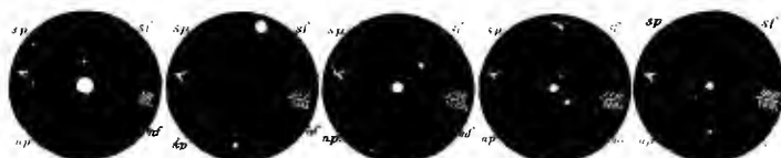
Rigel δ Orionis ε Orionis ζ Orionis λ Orionis
