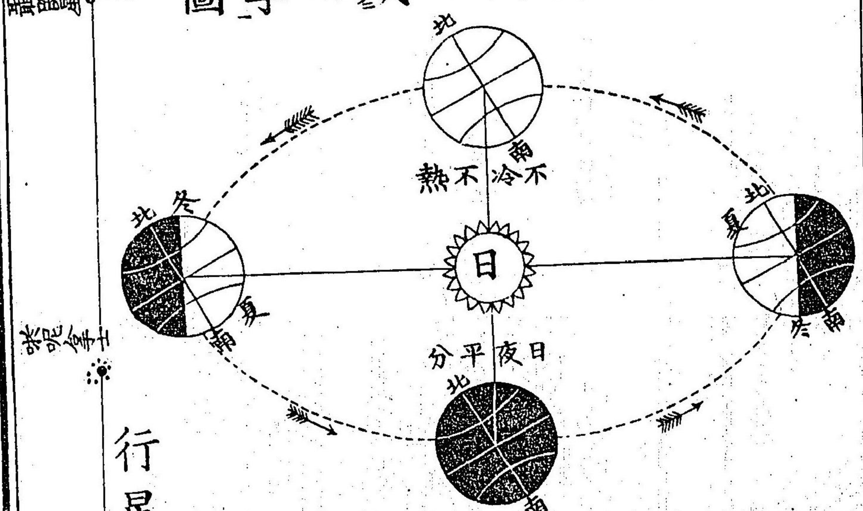
地球側倚圖四季圖
