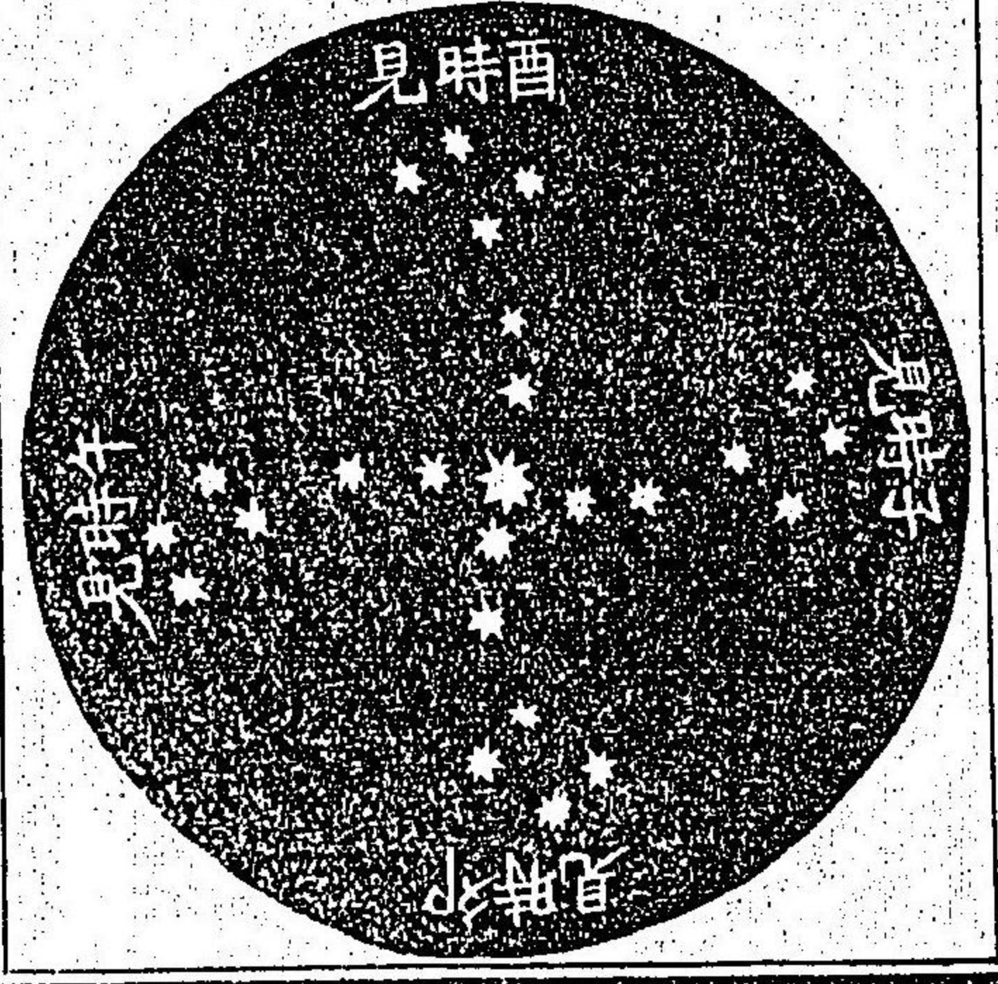
圖辰拱斗比
