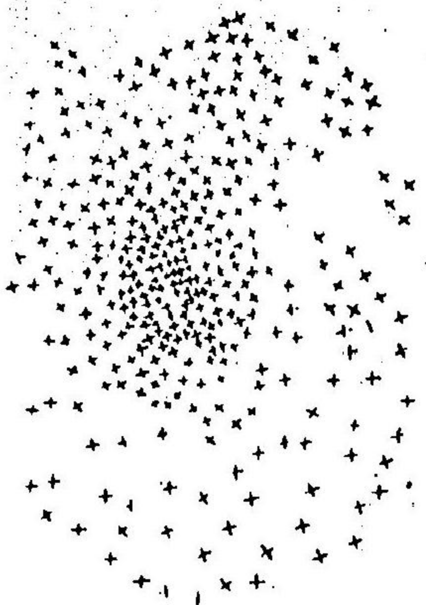
天河眾星圖
