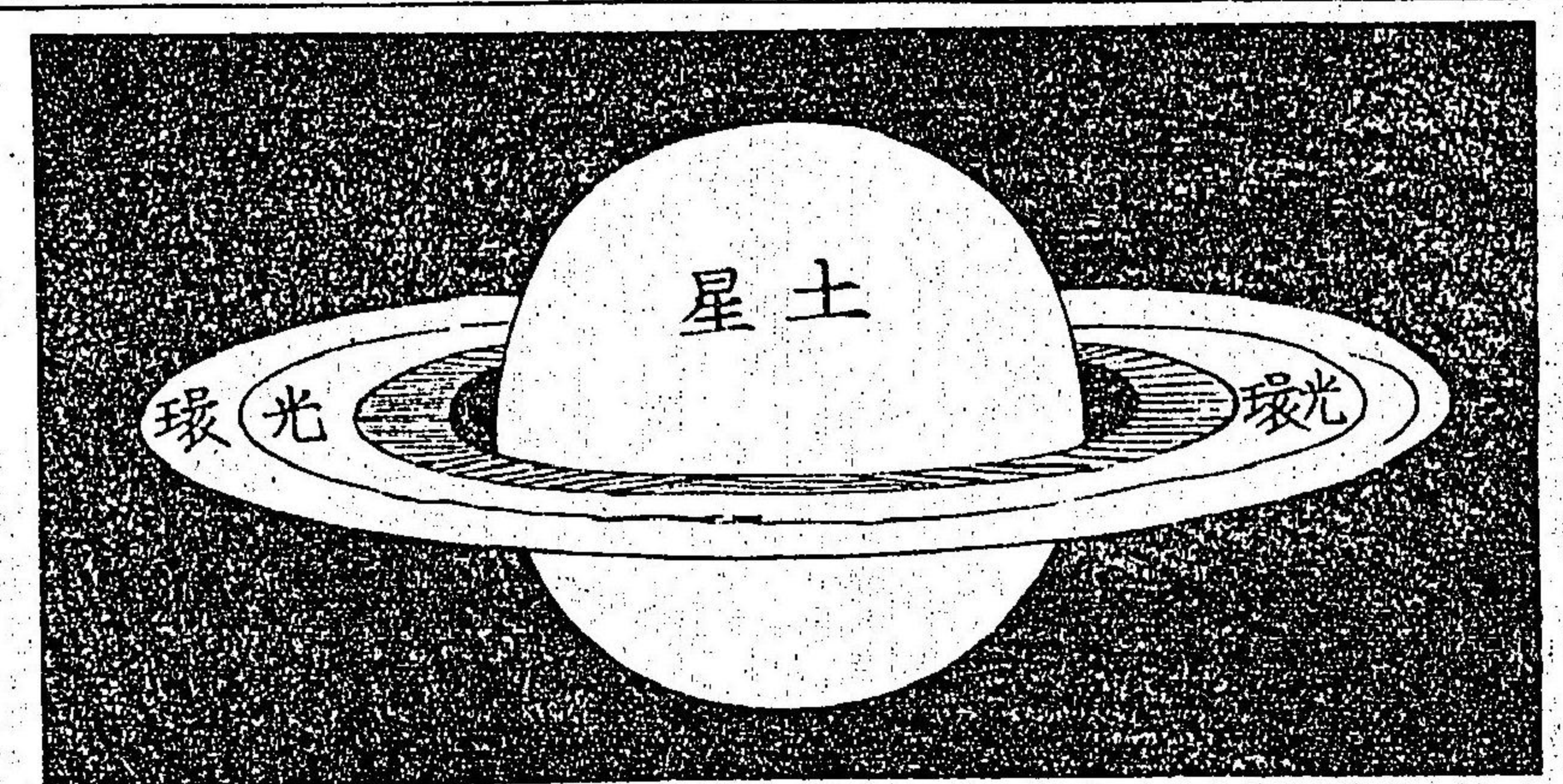
圖星土見平
