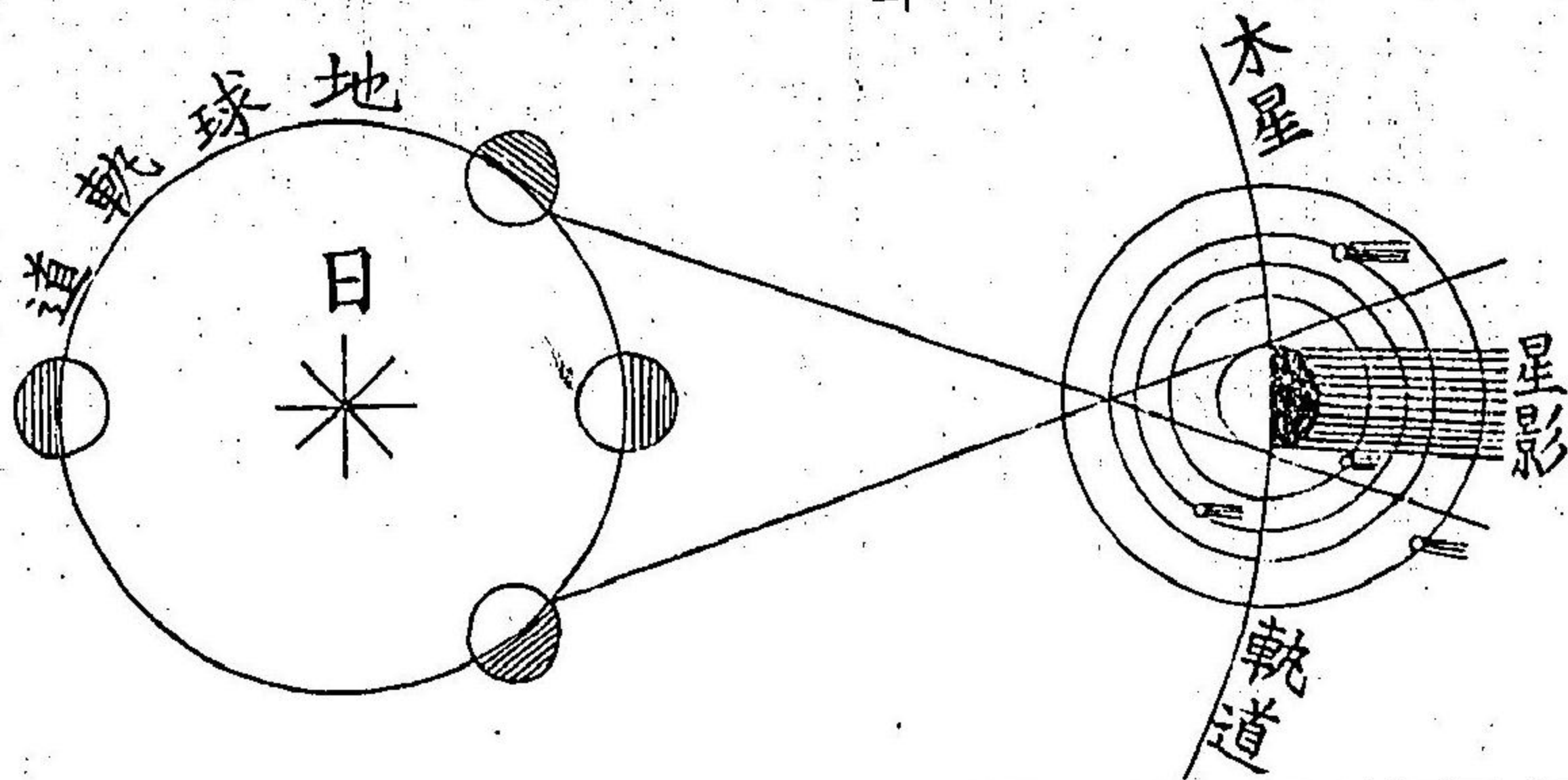
四小行星園木之星圖
