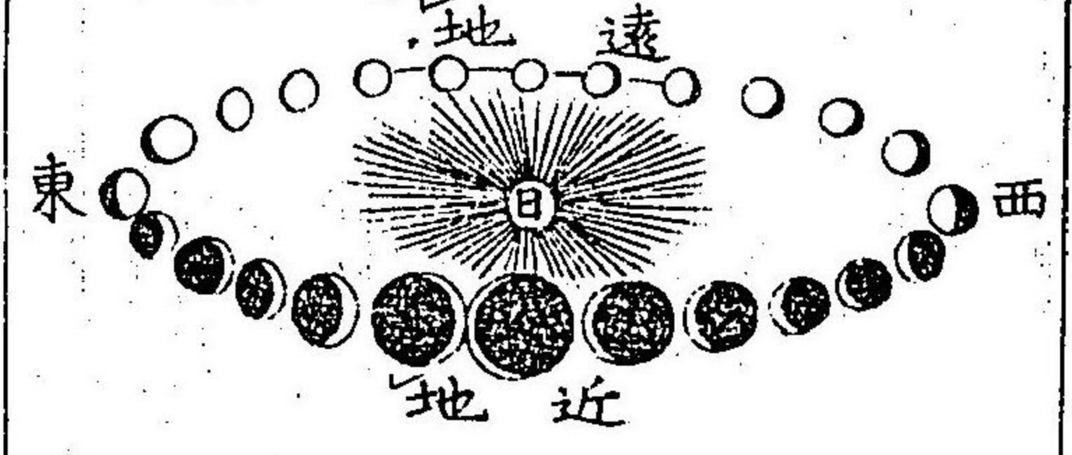
金星圓日行成盈缺之圖
