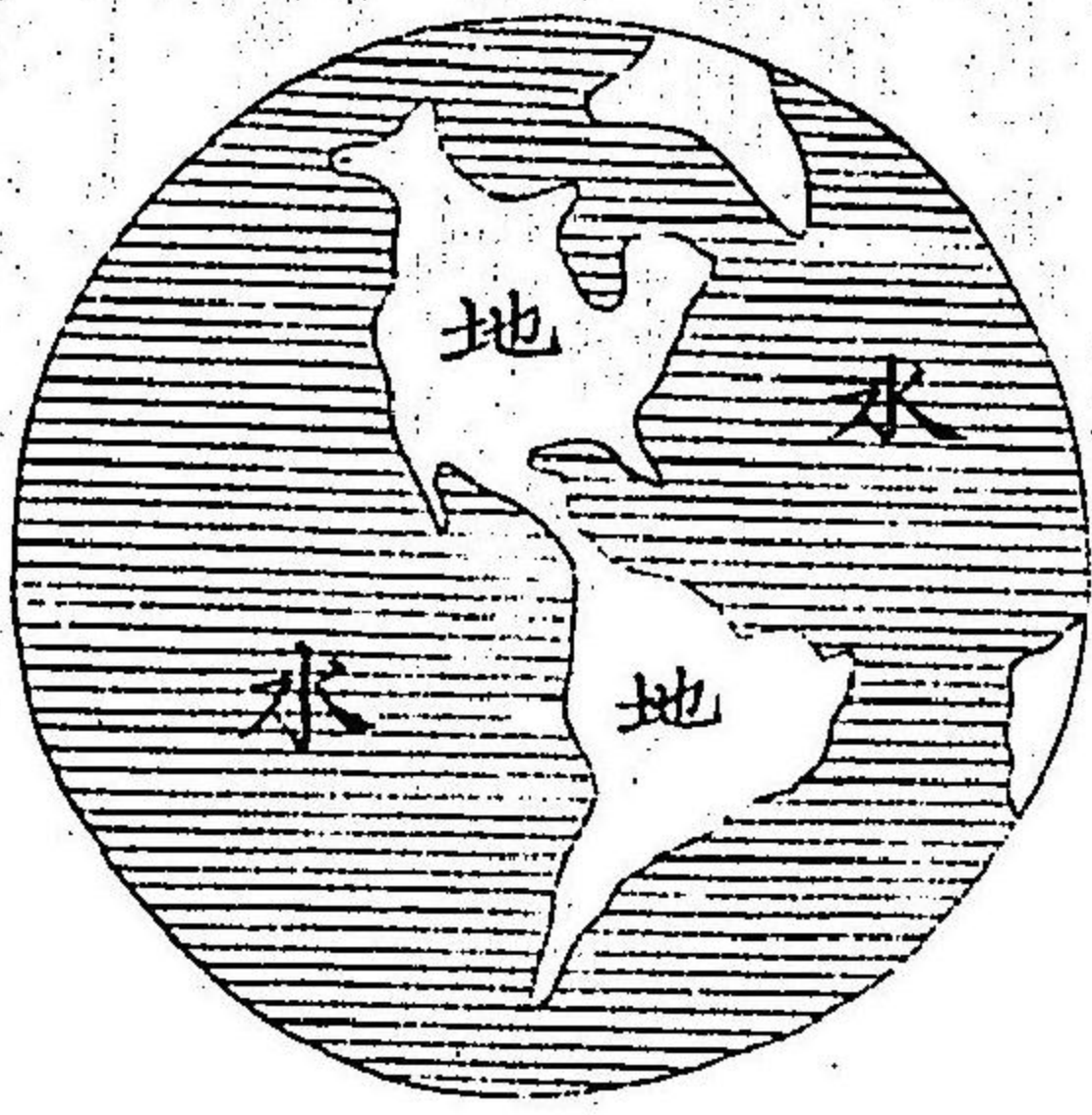
地球形像圖
